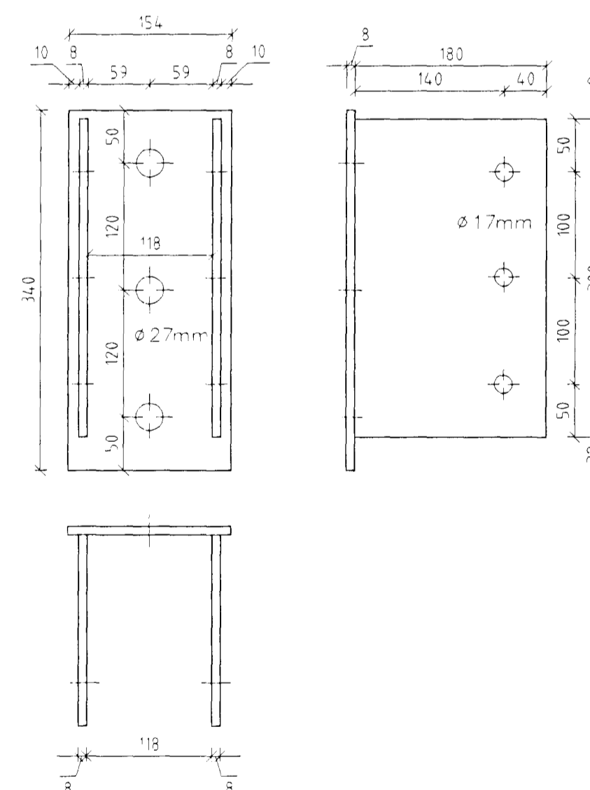
Stálfesting SF90 Mkv. 1:5 Samtals 3 stk
