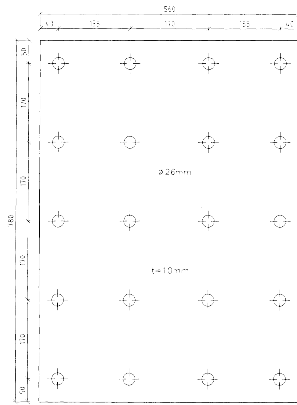
Stálfesting SF85 Mkv. 1:5 Samtals 6 stk
