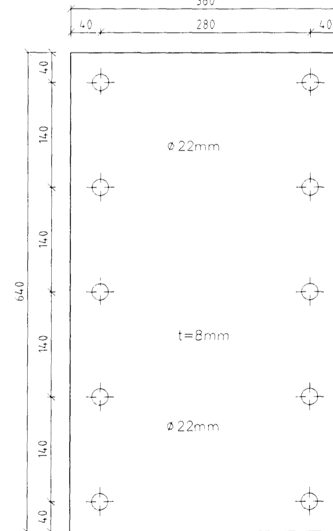
Stálfesting SF89.2 Mkv. 1:5 Samtals 6 stk
