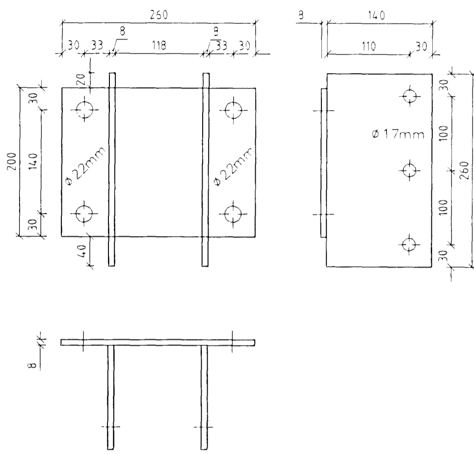
Stálfesting SF84 Mkv. 1:5 Samtals 254 stk
