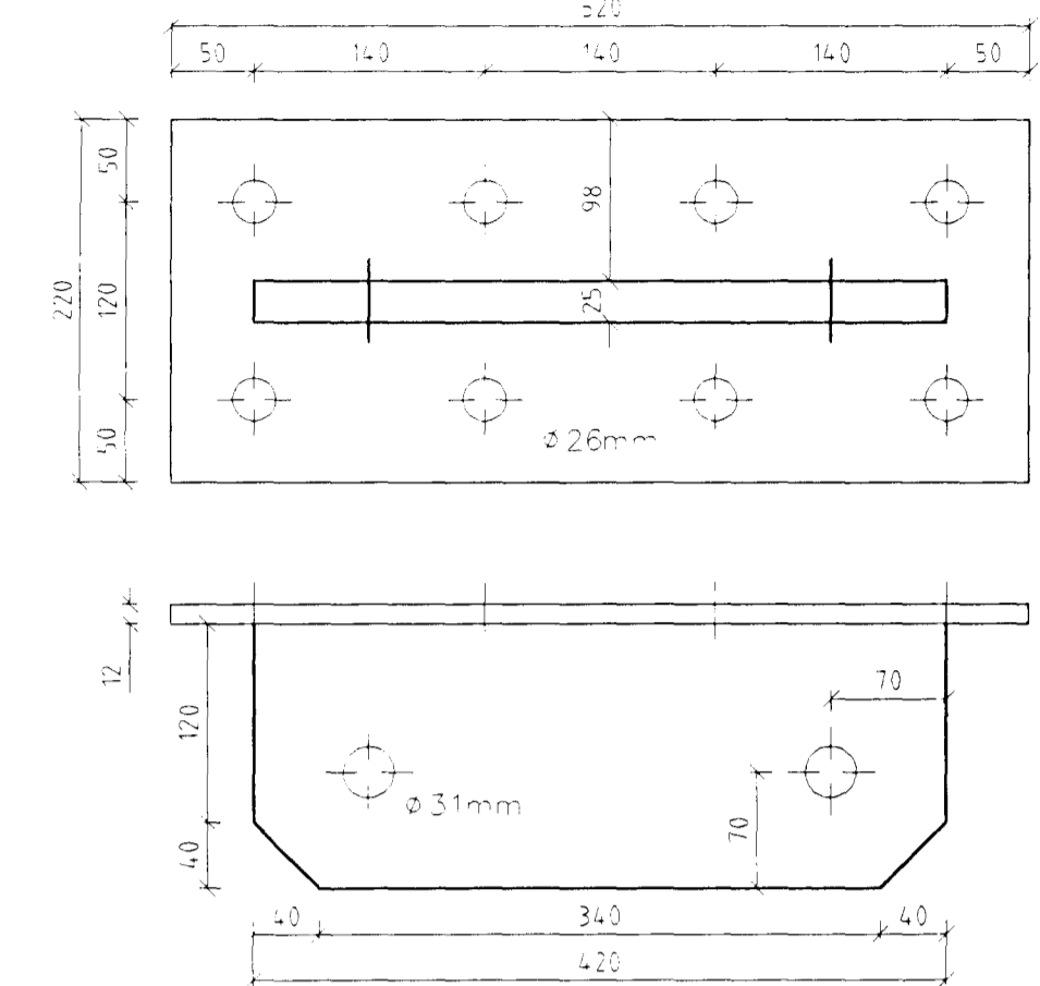
Stálfesting SF87 Mkv. 1:5 Samtals 3 stk
