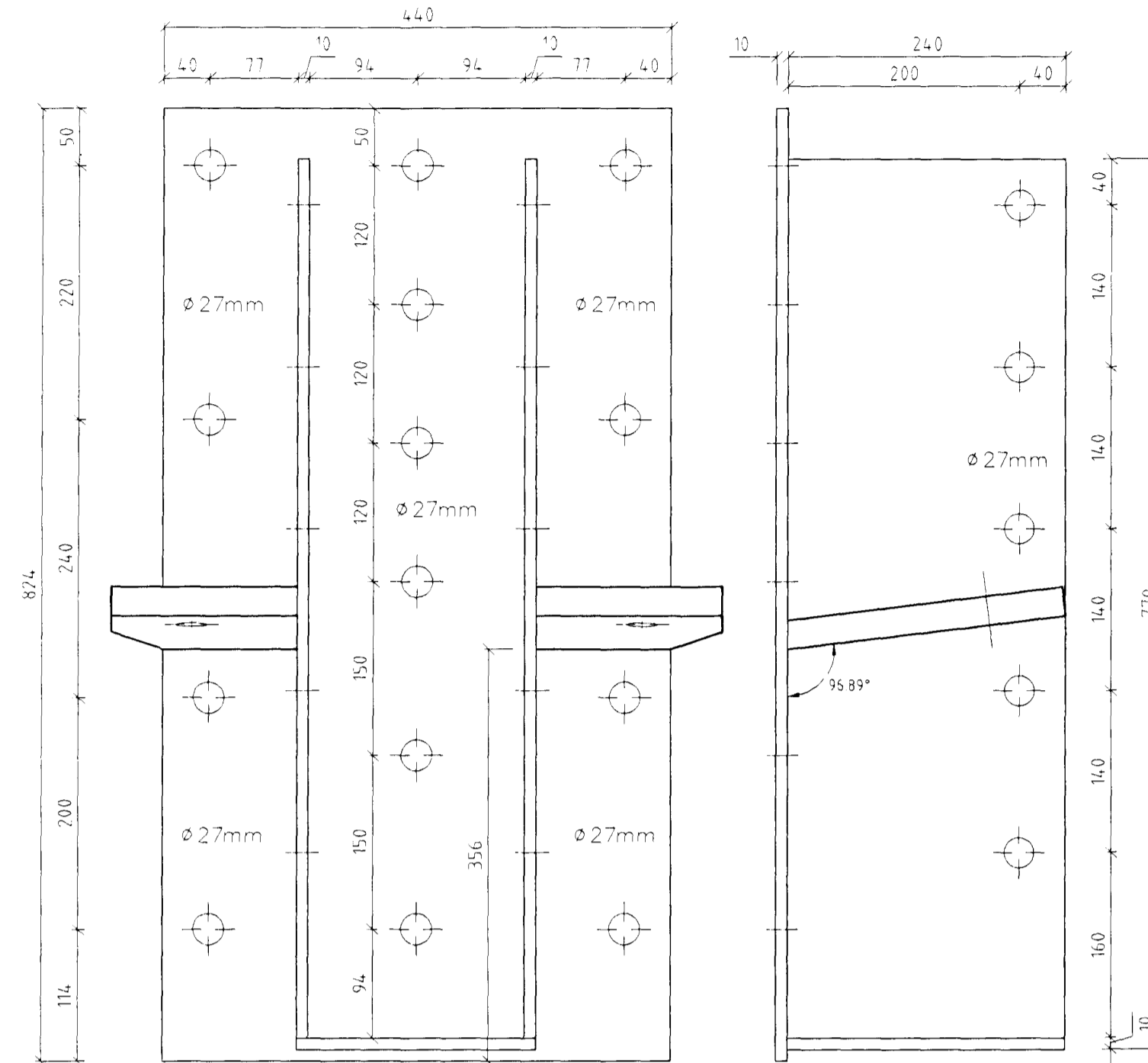
Stálfesting SF86 Mkv. 1:5 Samtals 3 stk
