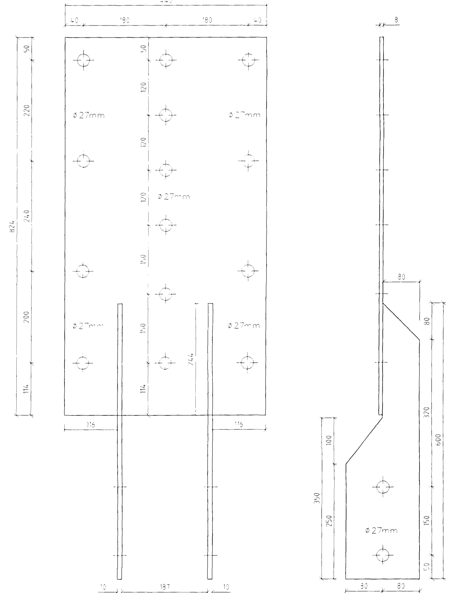
Stálfesting SF91 Mkv. 1:5 Samtals 3 stk
