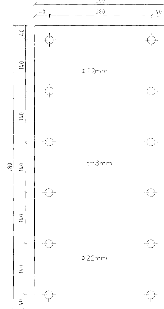
Stálfesting SF89.1 Mkv. 1:5 Samtals 2 stk
