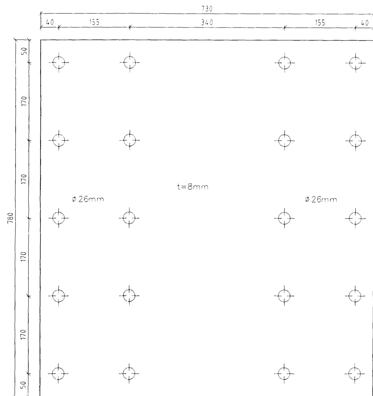
Stálfesting SF88 Mkv. 1:5 Samtals 2 stk
