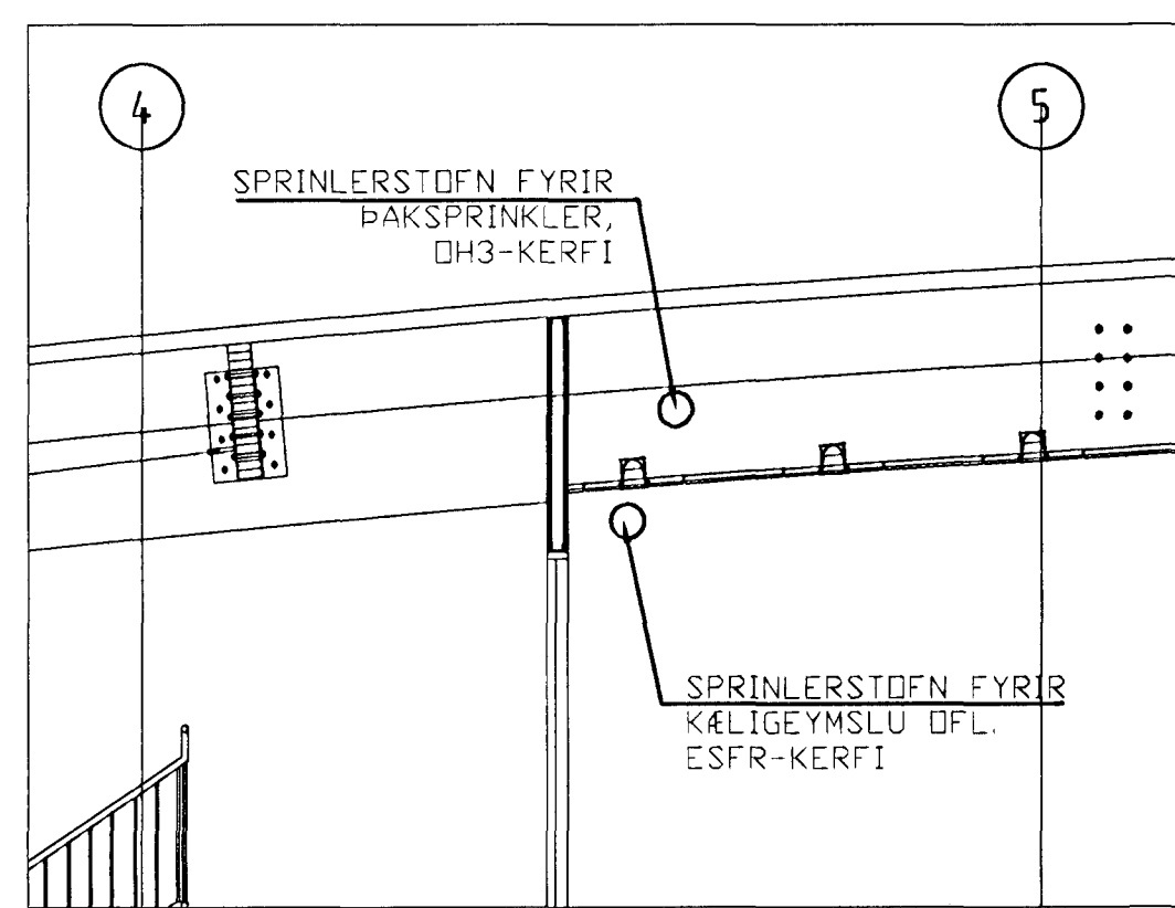
SNID Í SOFNLAGNIR SPRINKLERS, (KVARDI ENGINN)
