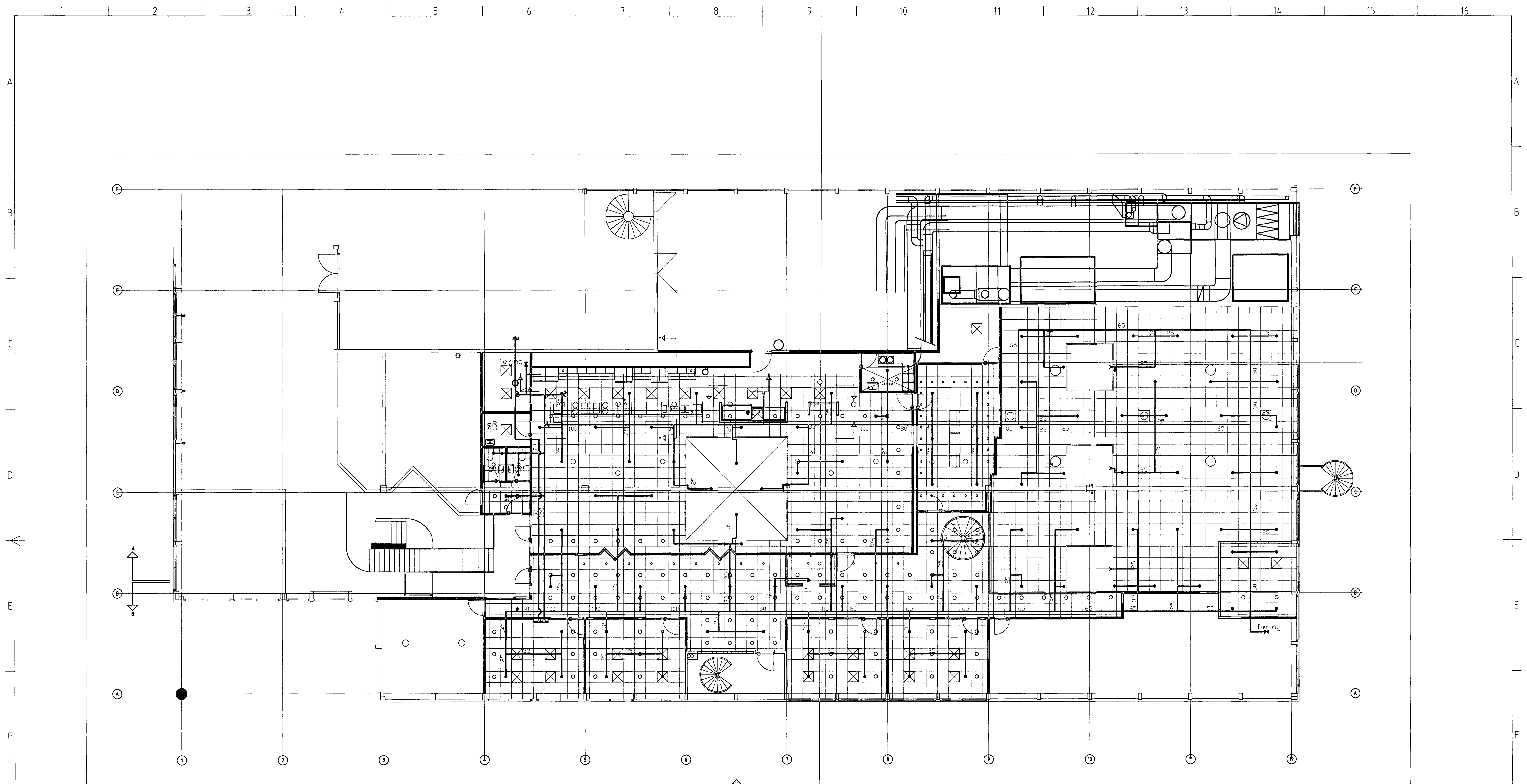
SNID Í SOFNLAGNIR SPRINKLERS, (KVARDI ENGINN)
