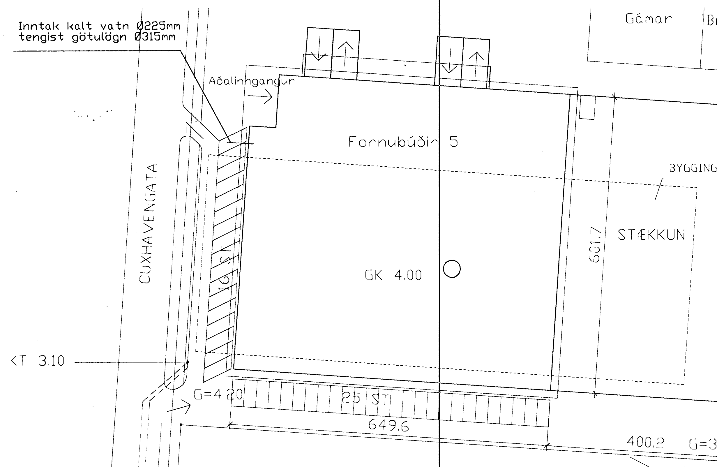
Afstöðumynd af inntaki
