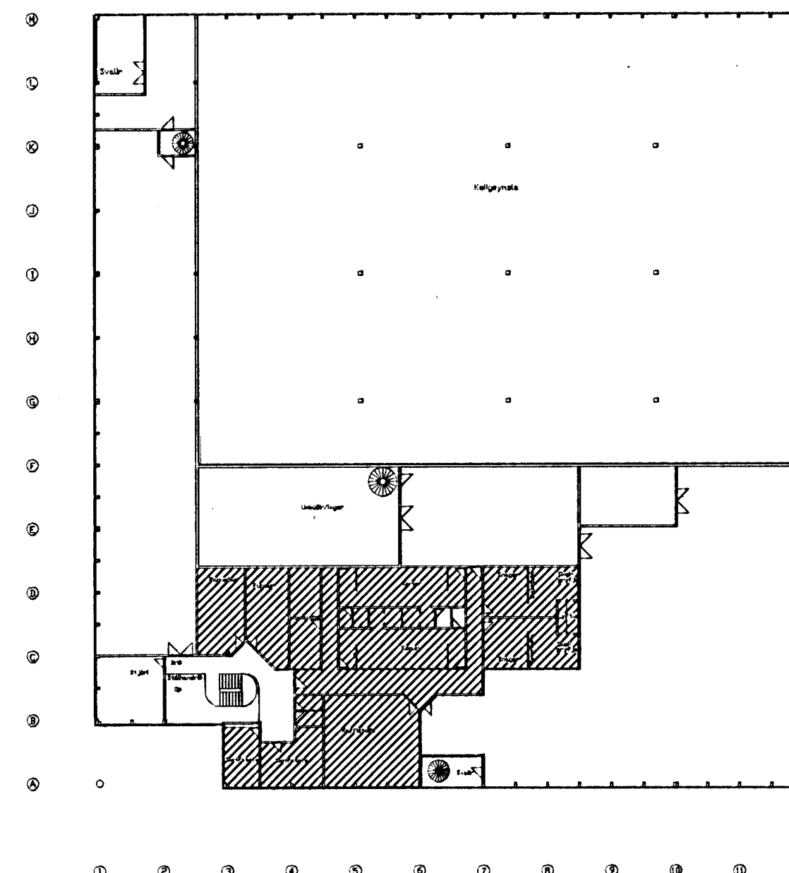
Sprinkler 2. hæðar (milliloft)
