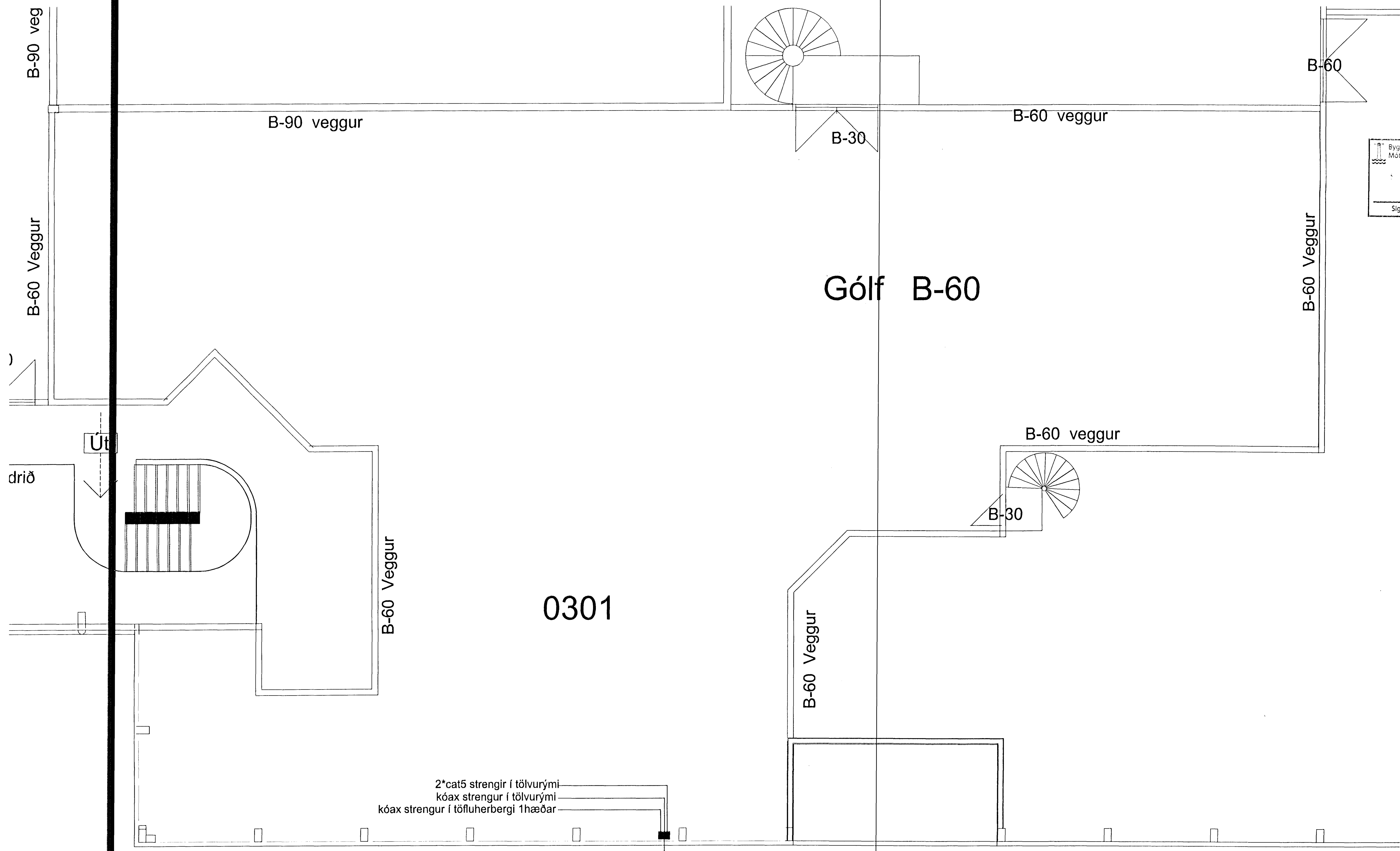
Grunnmynd geymsluloft 3. hæðar
