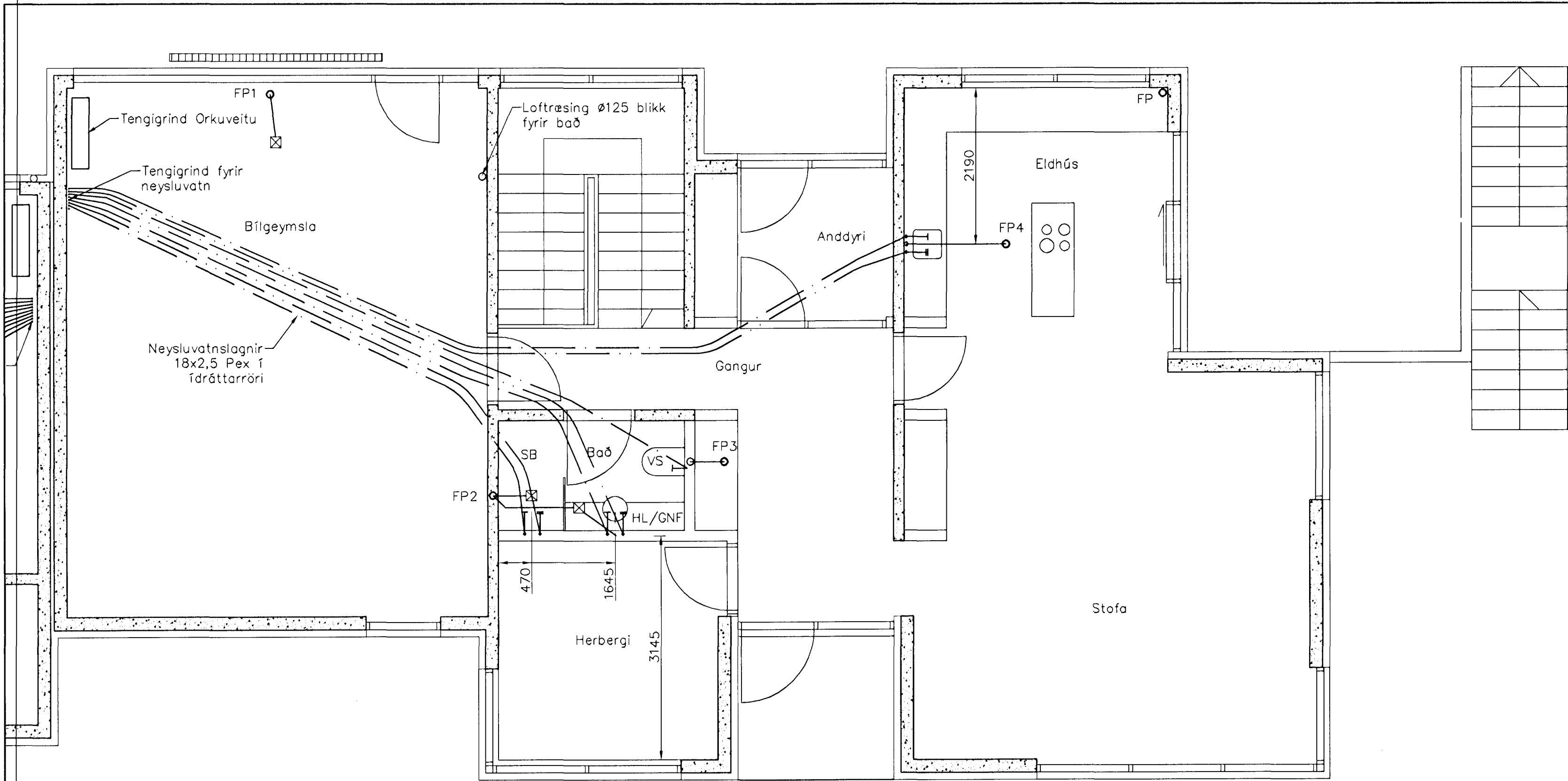
Neysluvatnslagnir 2. hæð, 1:50
