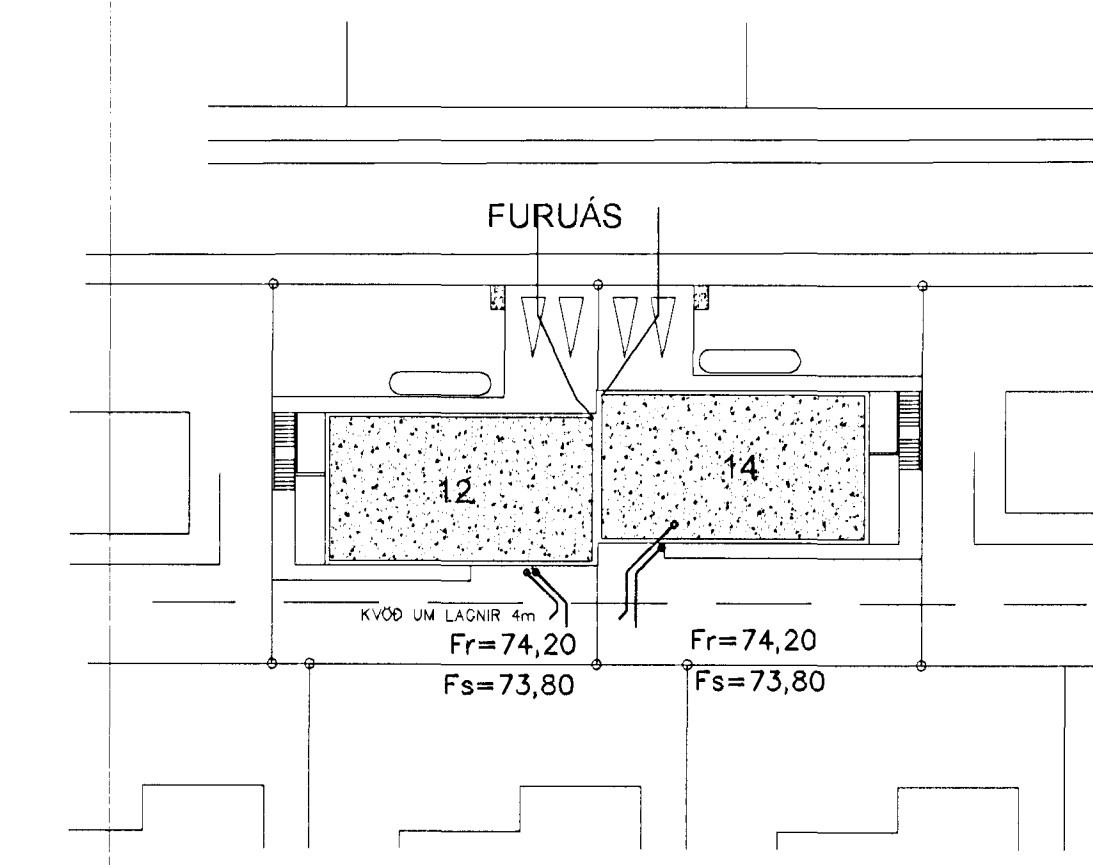
Afstöðumynd 1:500
