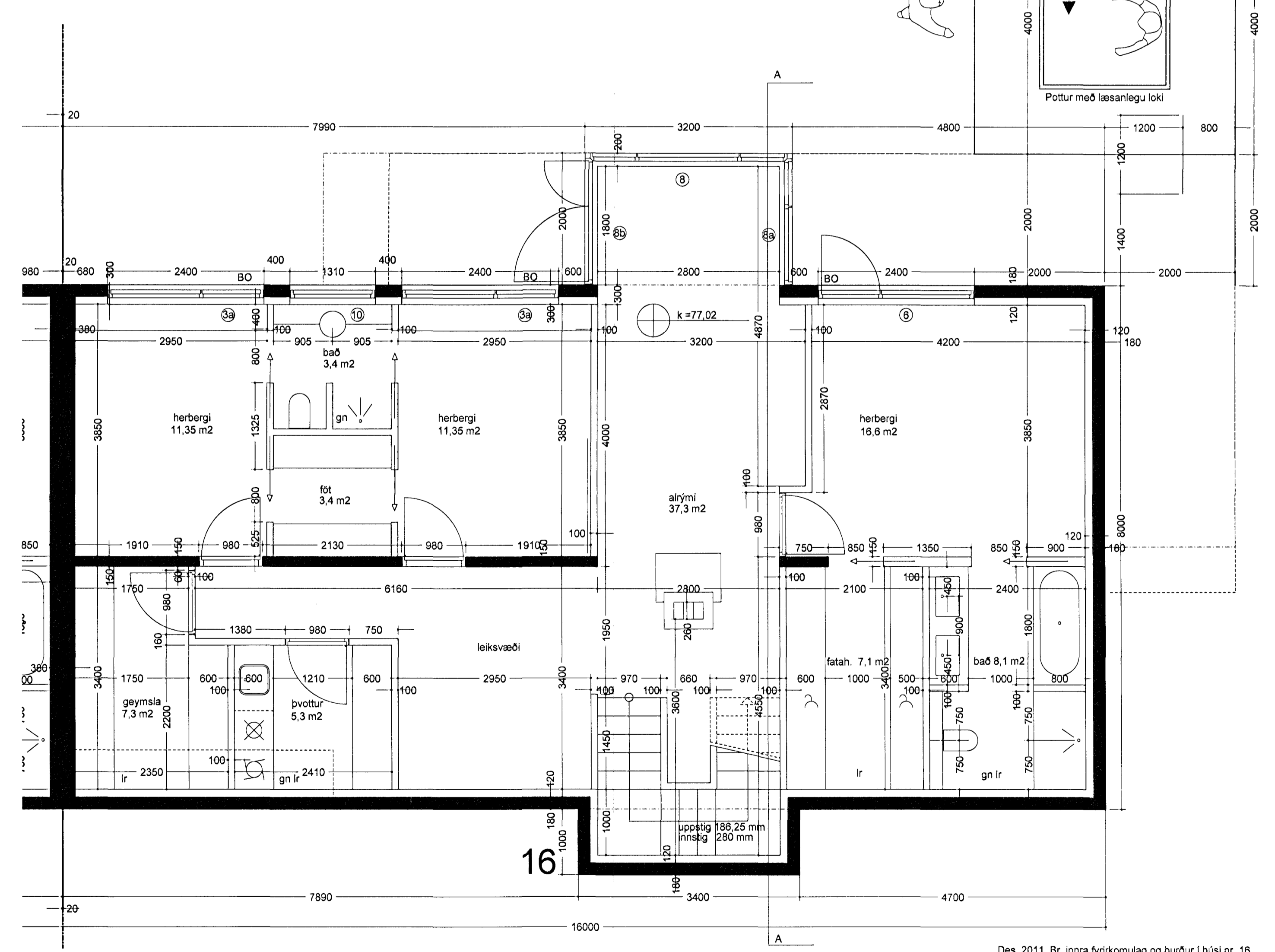
grunnmynd neðri hæðar
