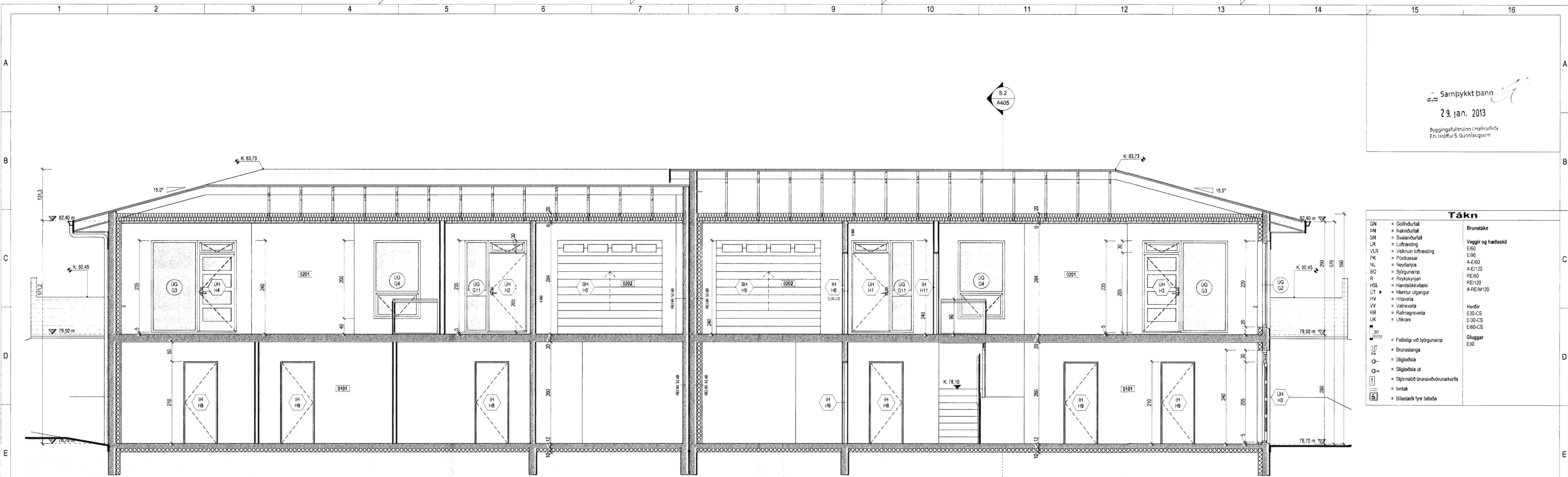
Snið S.1 1:50
