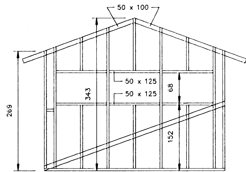
NORÐURHLIÐ, M=1:50
