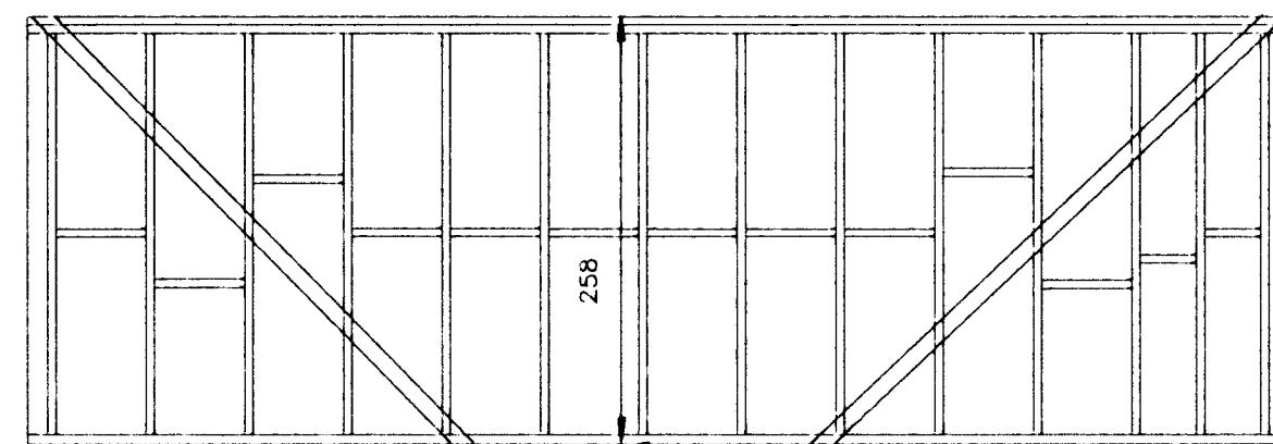
VESTURHLIÐ, M=1:50
