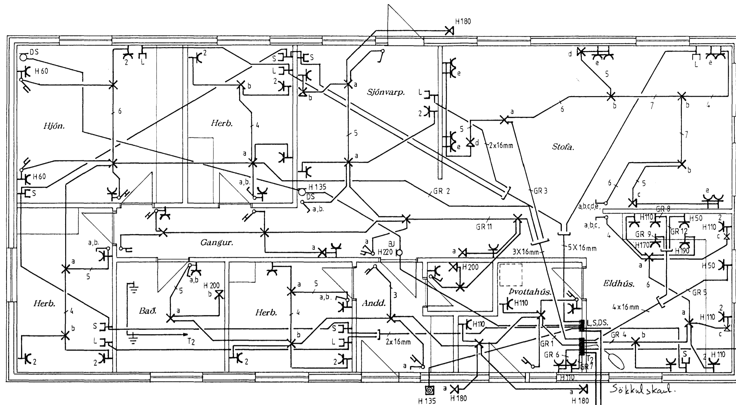
Grunnmynd Mkw 1:50.
