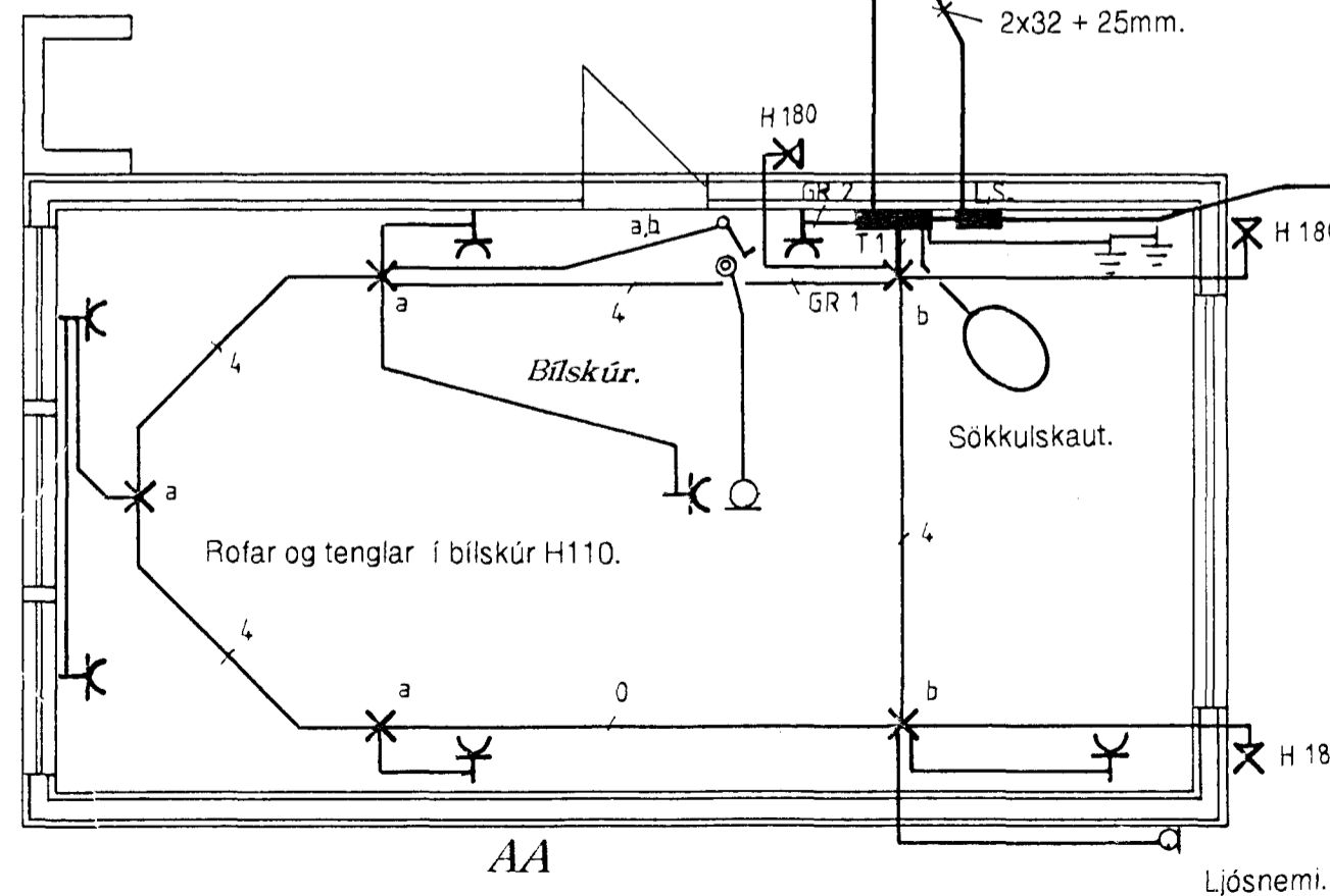
Bílskúr Mkw 1:50.
