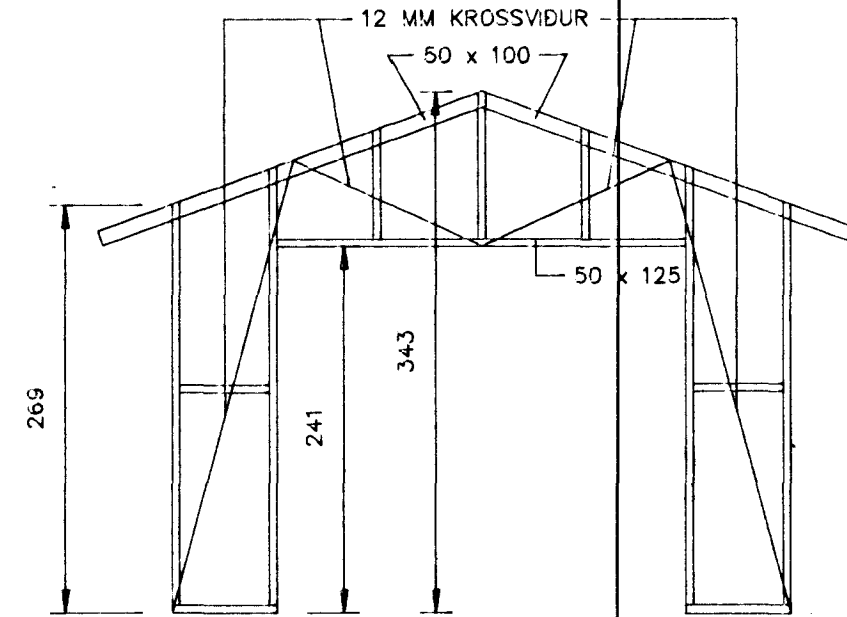
SUÐURHLID, M=1:50
