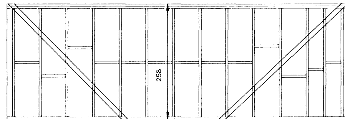
VESTURHLID, M=1:50
