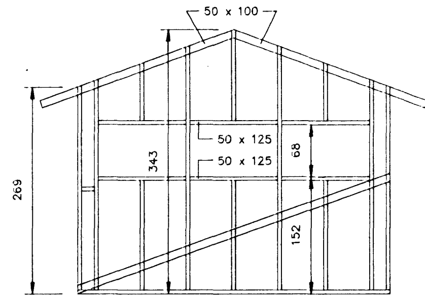
NORÐURHLID, M=1:50
