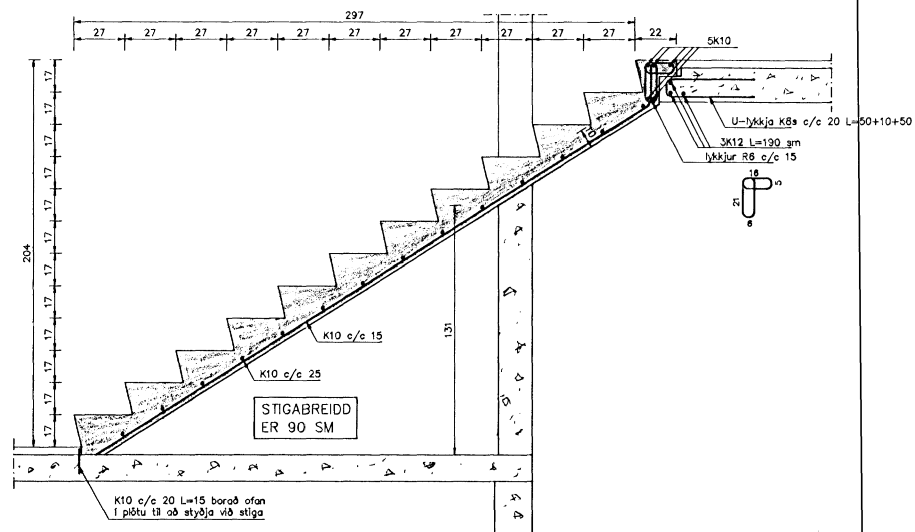
Stigi á milli hæða snið mkv. 1:20
