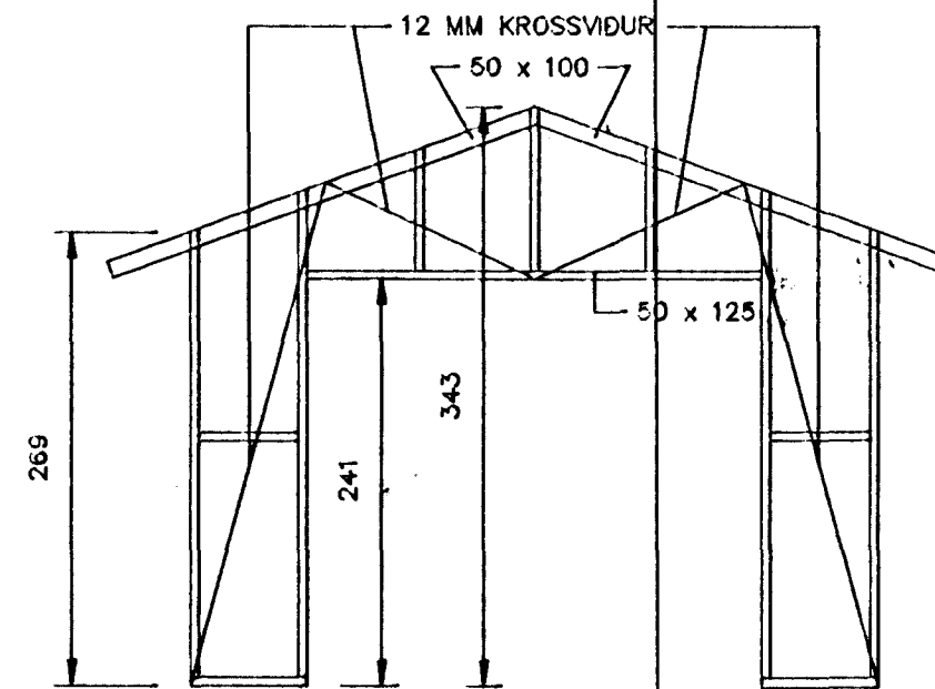
SUÐURHLIÐ, M=1:50
