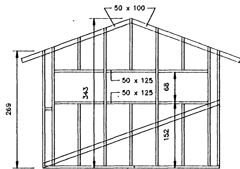
NORÐURHLIÐ, M=1:50
