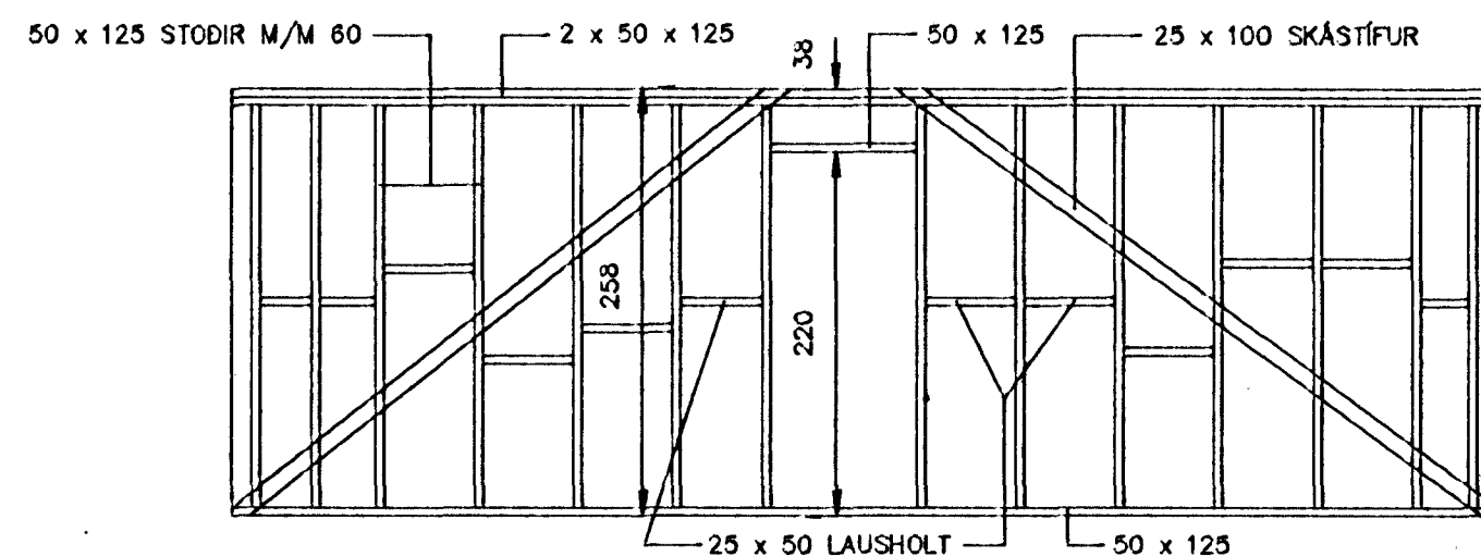
AUSTURHLIÐ, M=1:50
