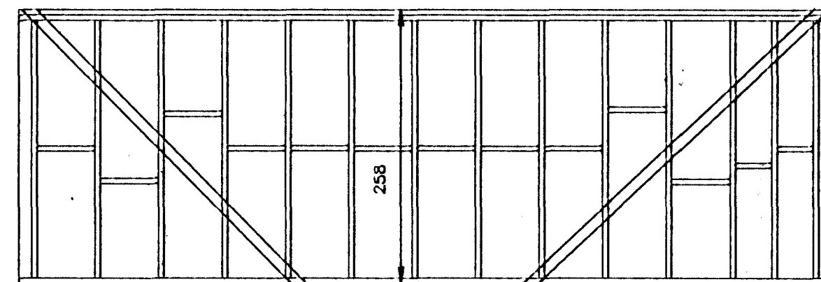
VESTURHLIÐ, M=1:50
