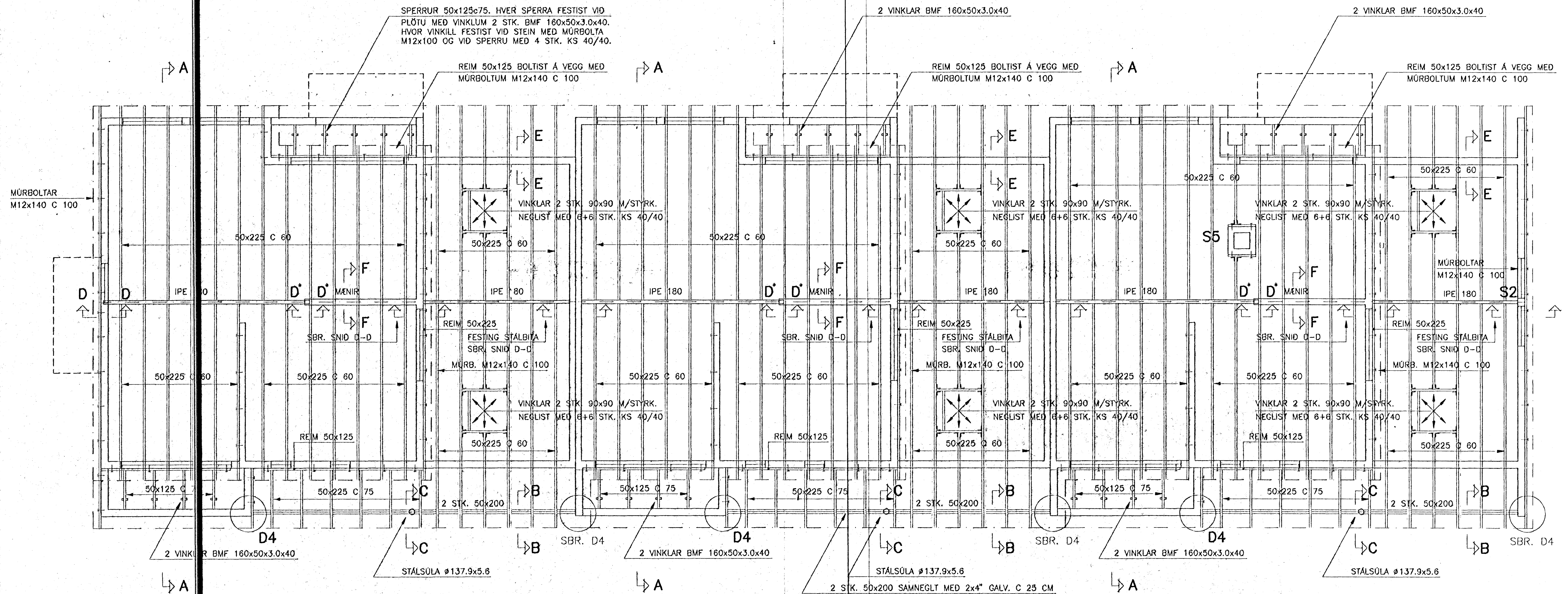
GRUNNMYND ÞAKS 1:50
