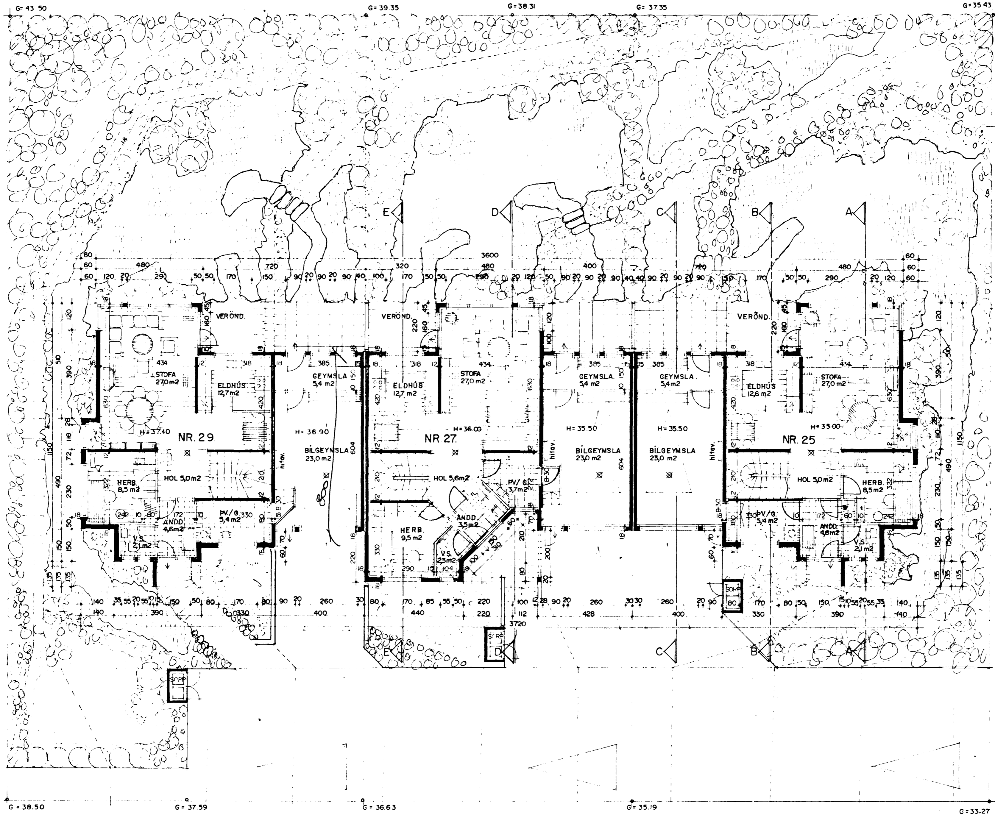
GRUNNMYND I. HÆÐAR. MKV. 1:100.
