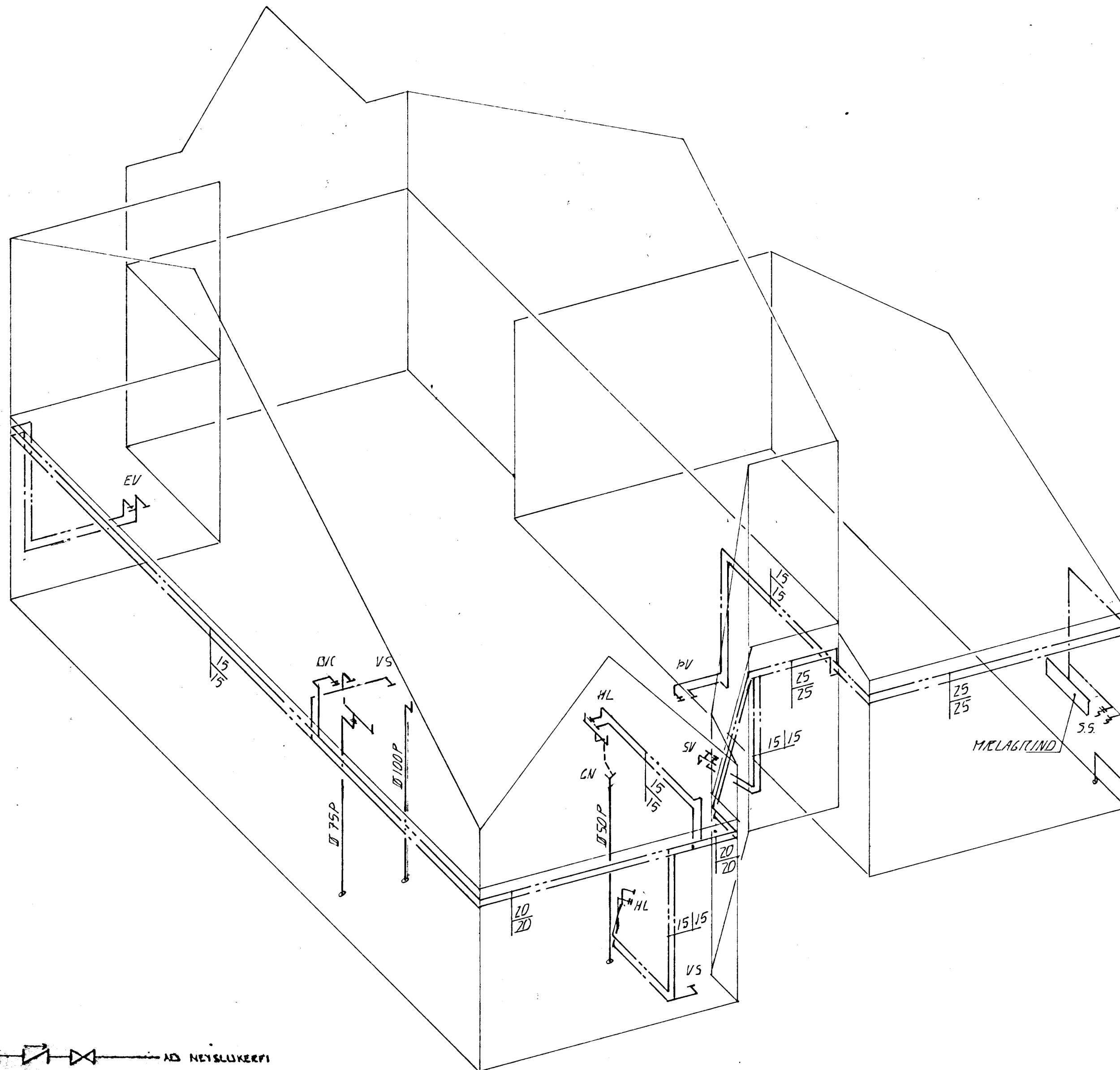
VATNSLAGNIR. RÚMMYND. 1:50
