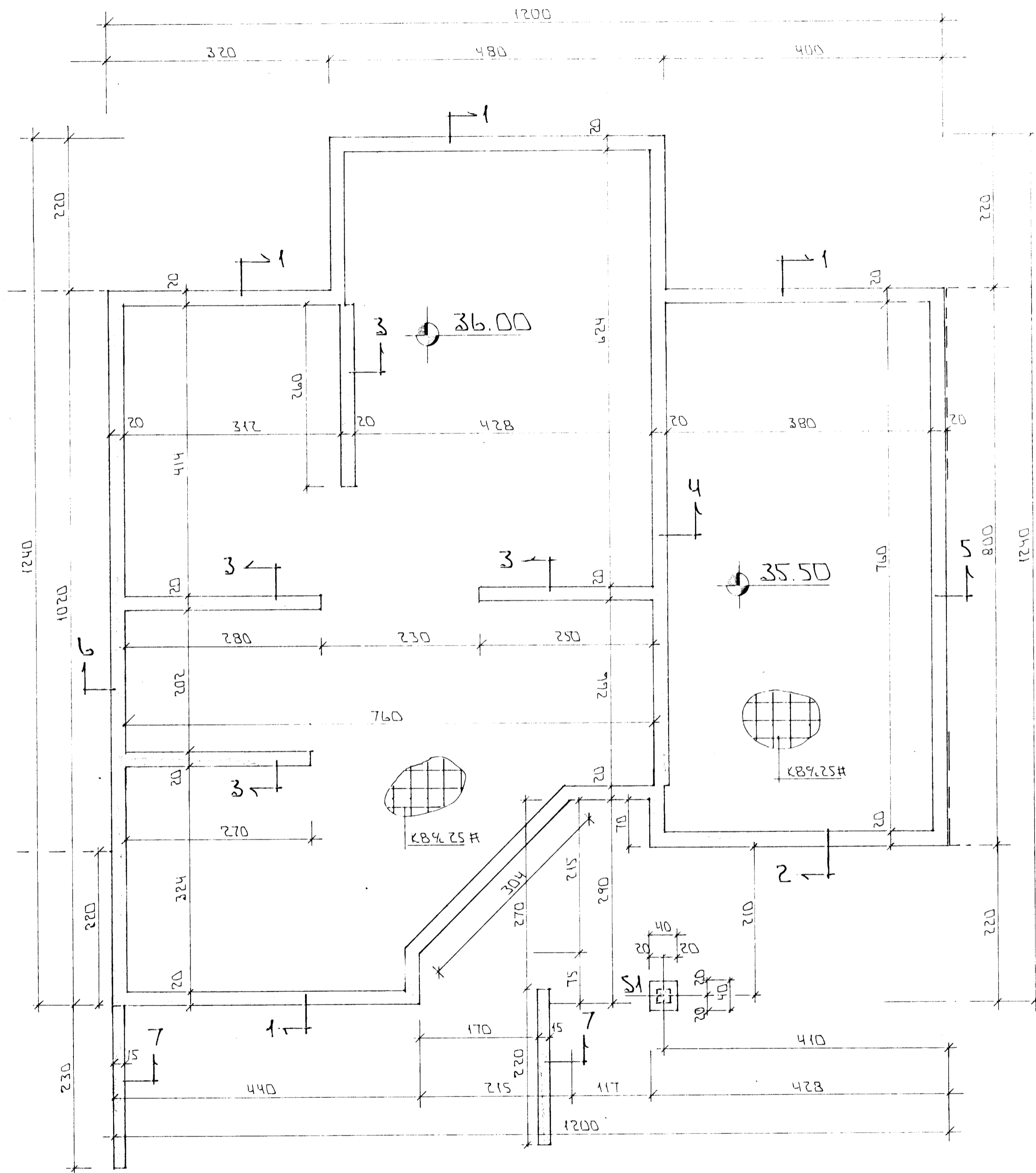
GRUNNMÝND 1:50
