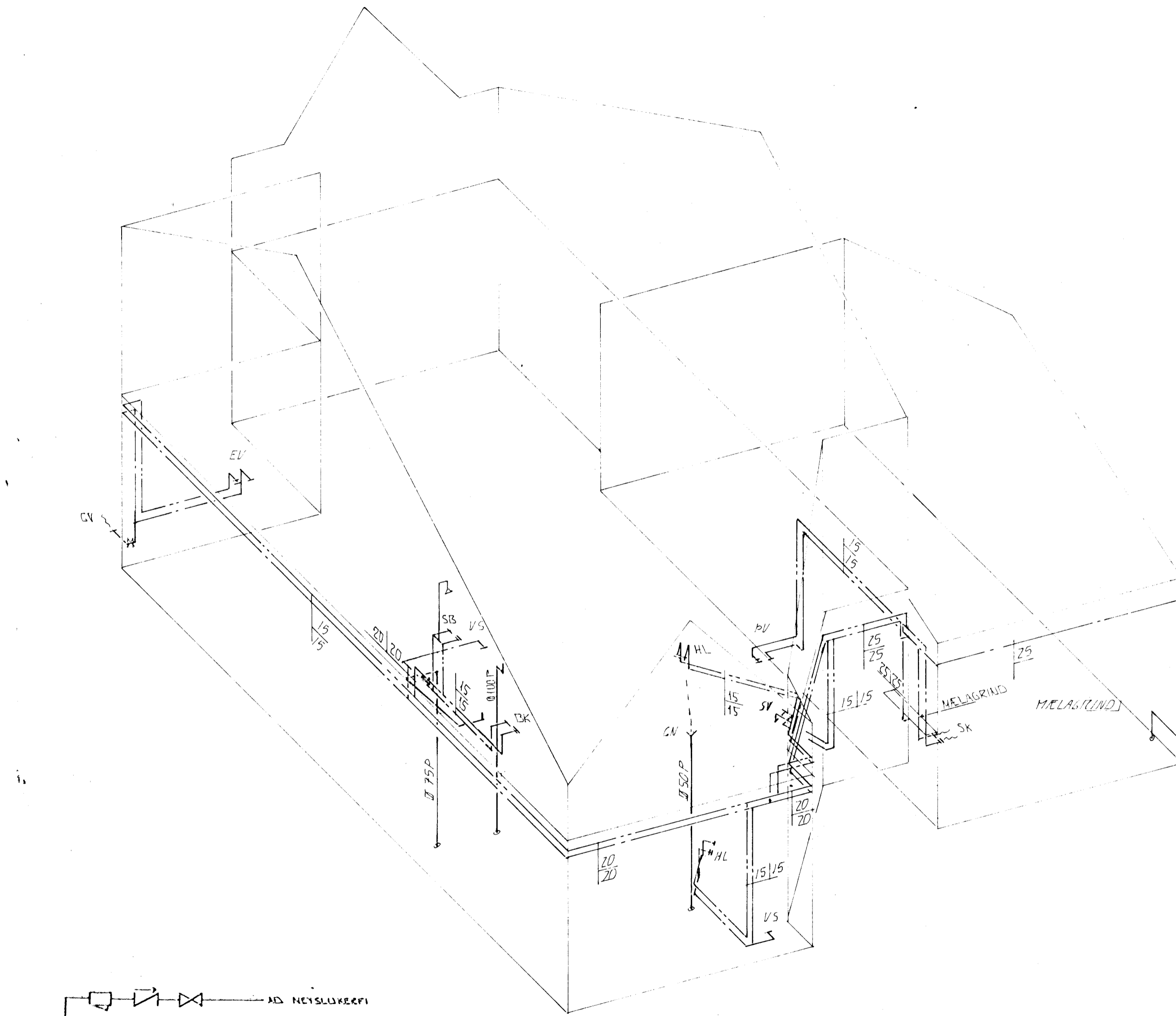
VATNSLAGNIR. RÚMMYND. 1:50
