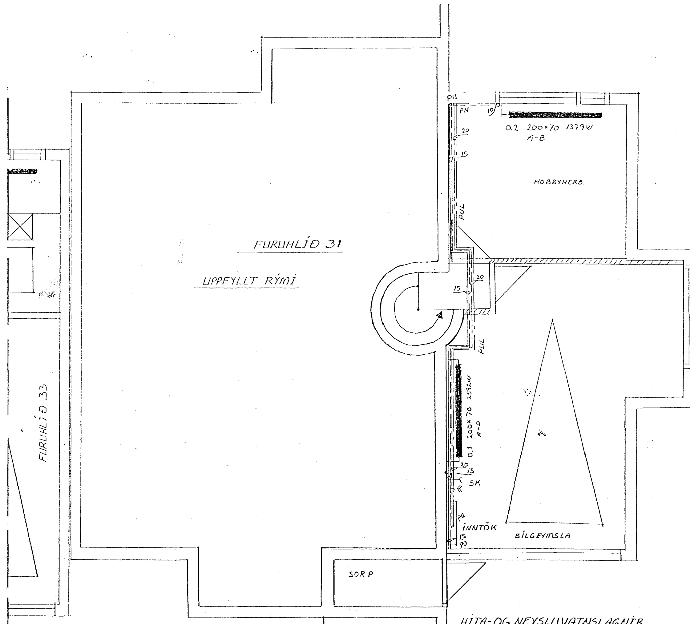
HITA- OG NEYSLUVATNSLAGNIR GRUNNMYND 1. HÆÐAR. MKV.: 1:50
