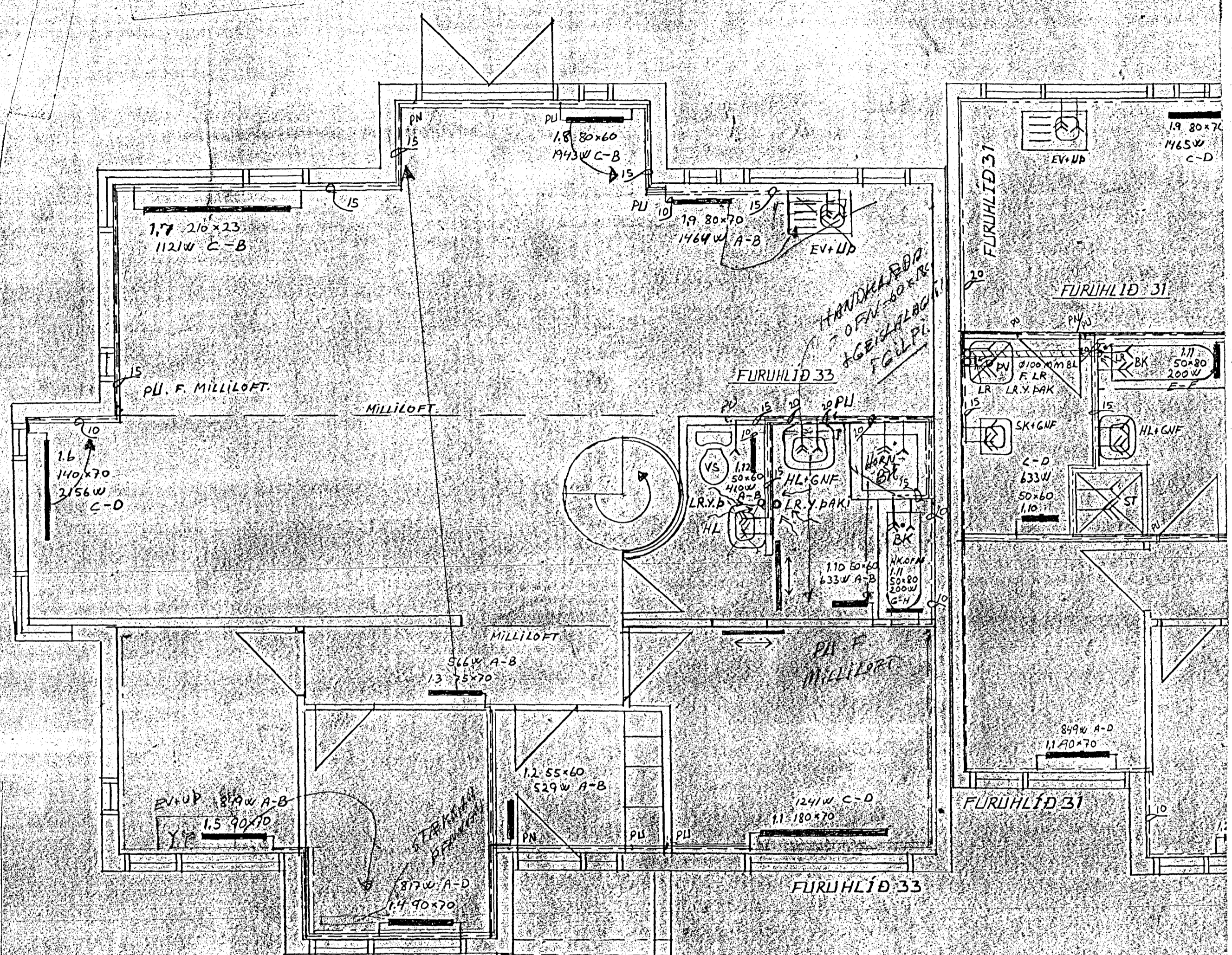
HITA- OG NEYSLUVATNSLAGNIR GRUNNMYND 2. HEDAR MKV.: 1:50
