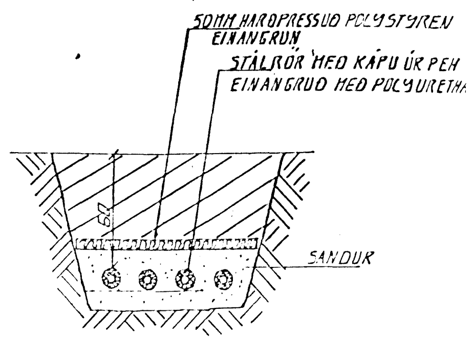
SNIÐ 1:1-20 LAGNIR Í JÖRÐ
