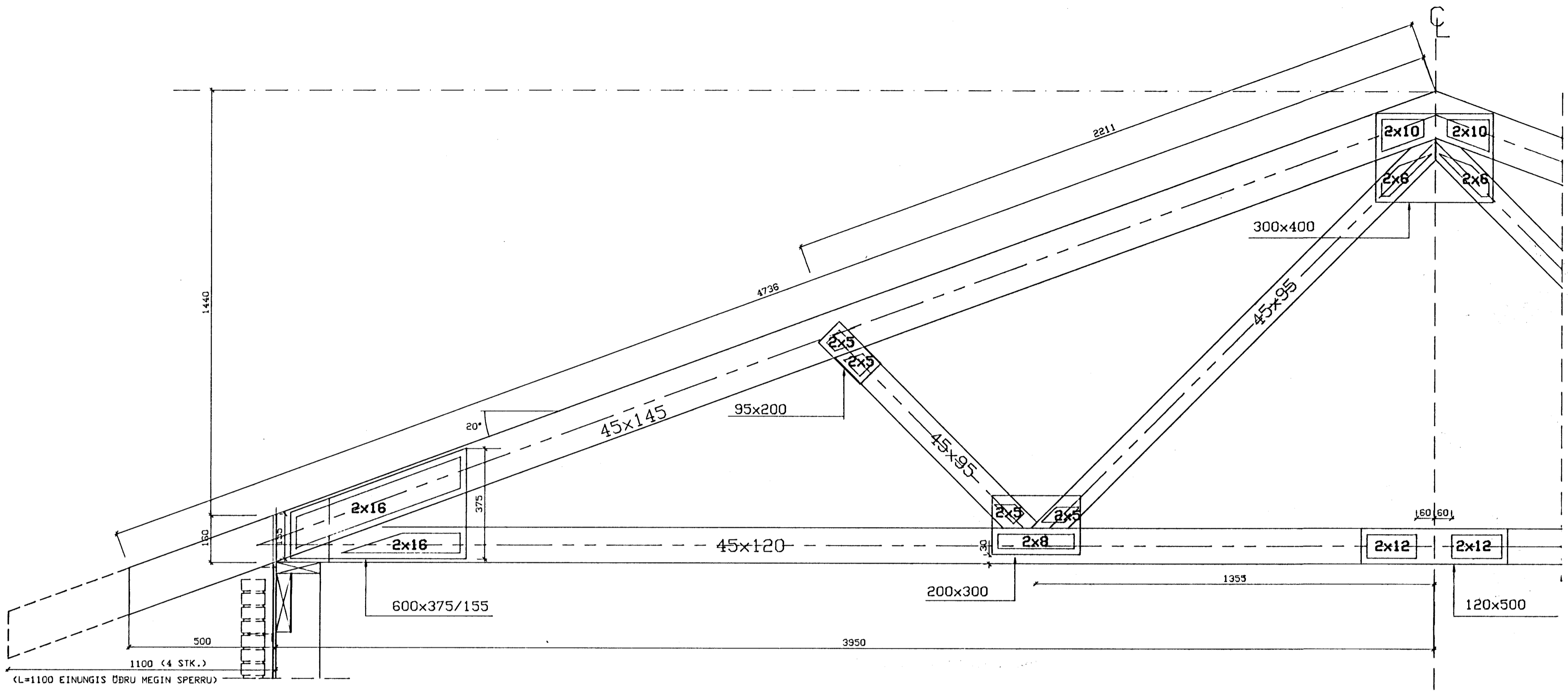
KRAFTSPERRA 1:10 L=7.9 M
