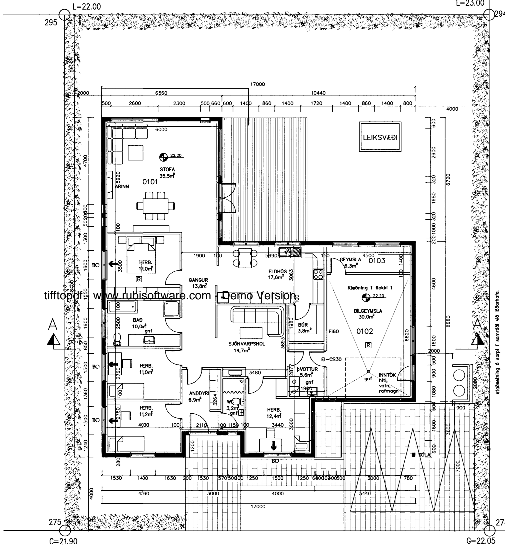
GRUNNMYND 1:100
