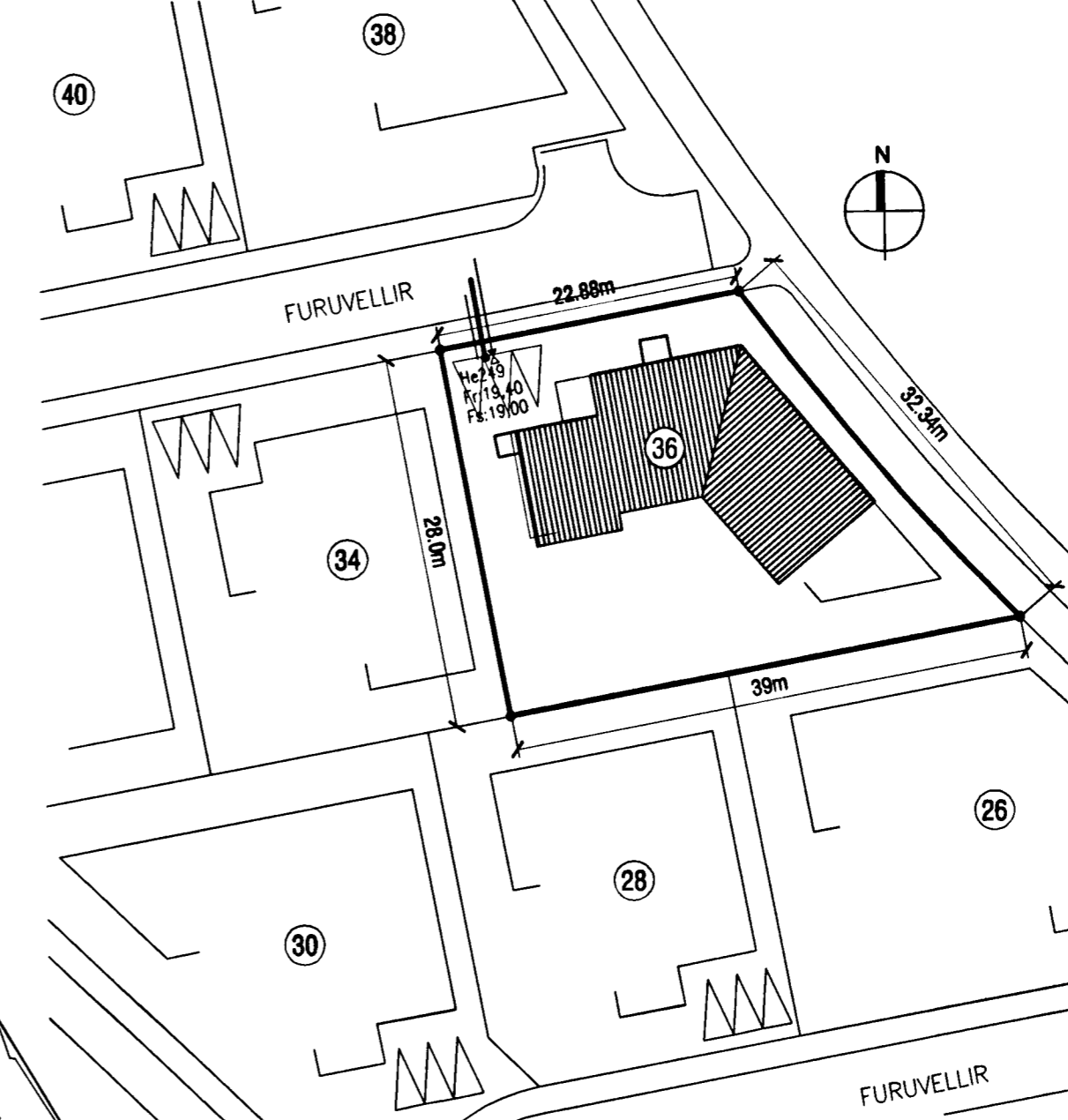
AFSTÖÐUMYND mkv. 1:500
