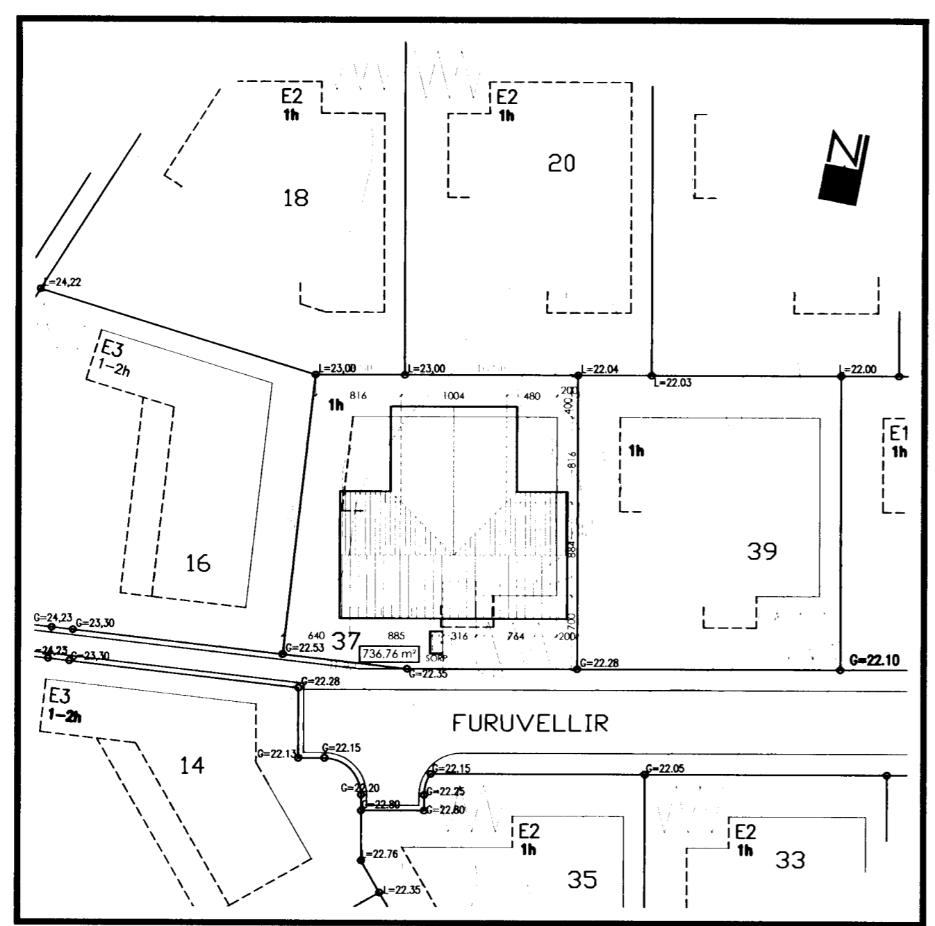
afstöðumynd 1:500
