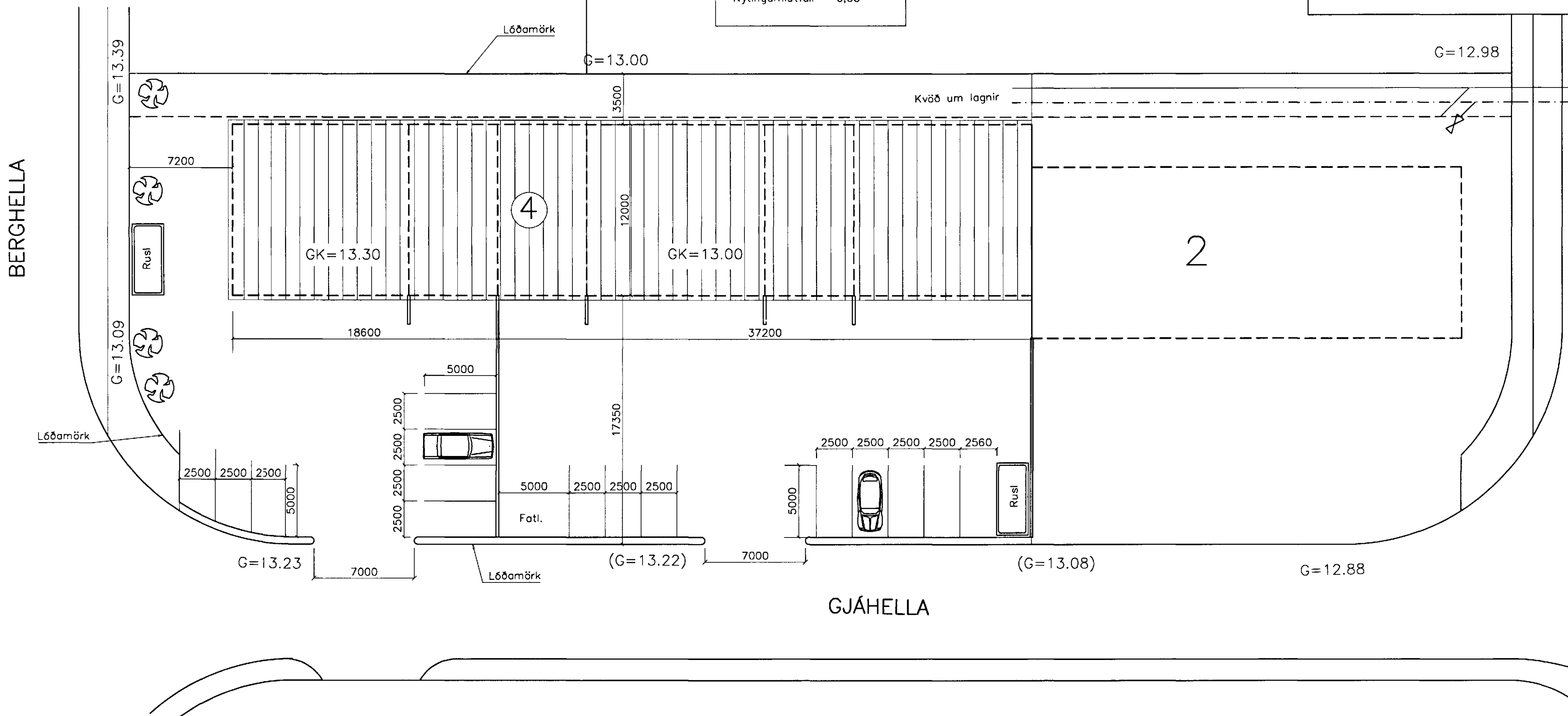
Grunnmynd lóðar, 1:200
