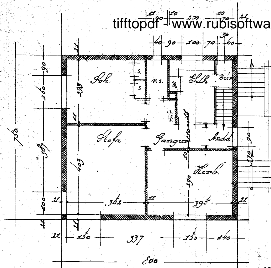
1. hæðin
