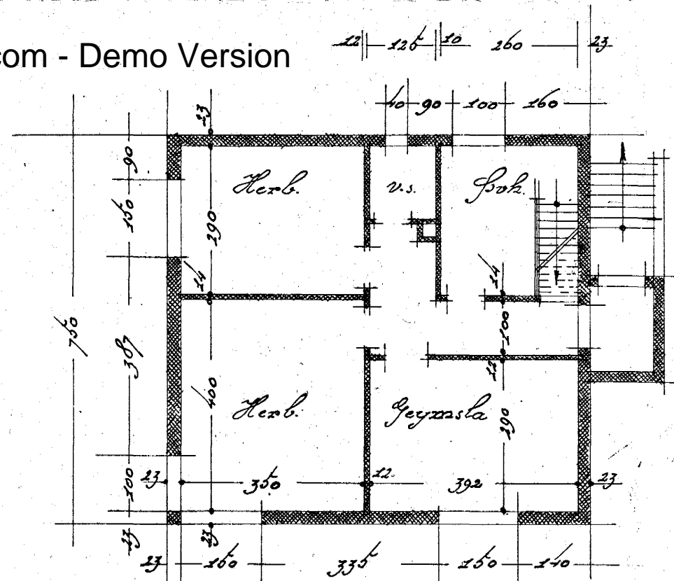
2. hæðin
