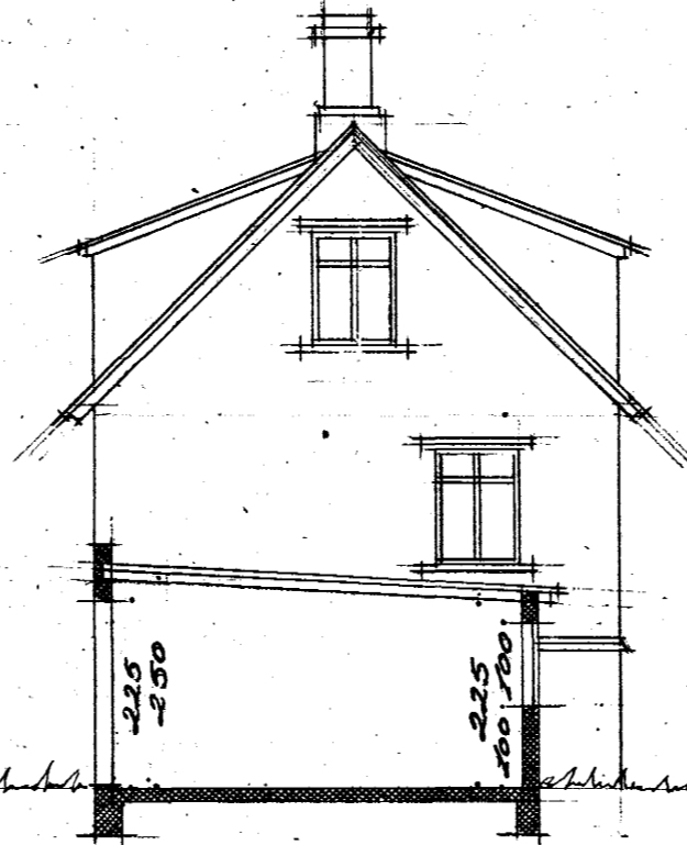
Sneiðing
