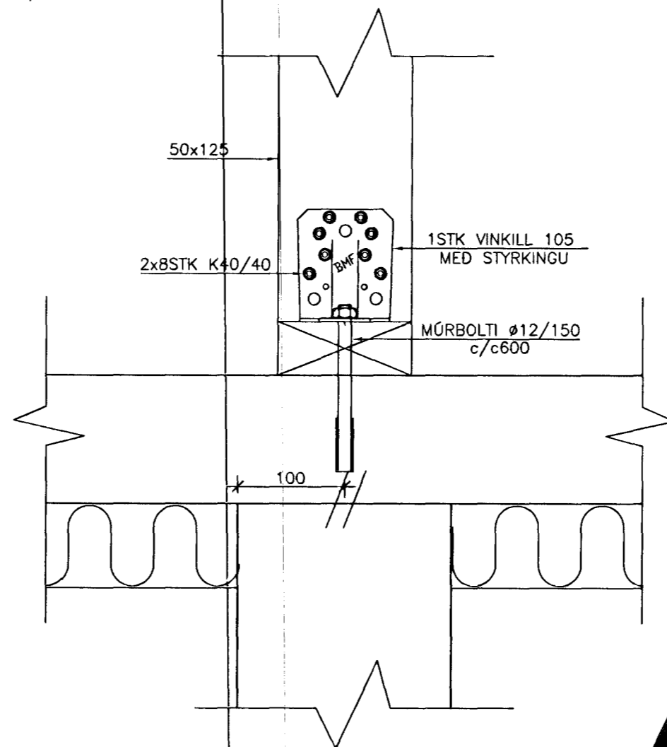
SNIÐ 12 1/5 B02&03
