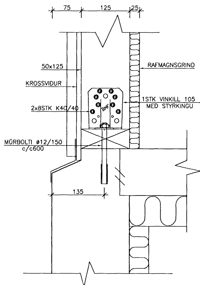
SNIÐ 10 1/5 B02&03
