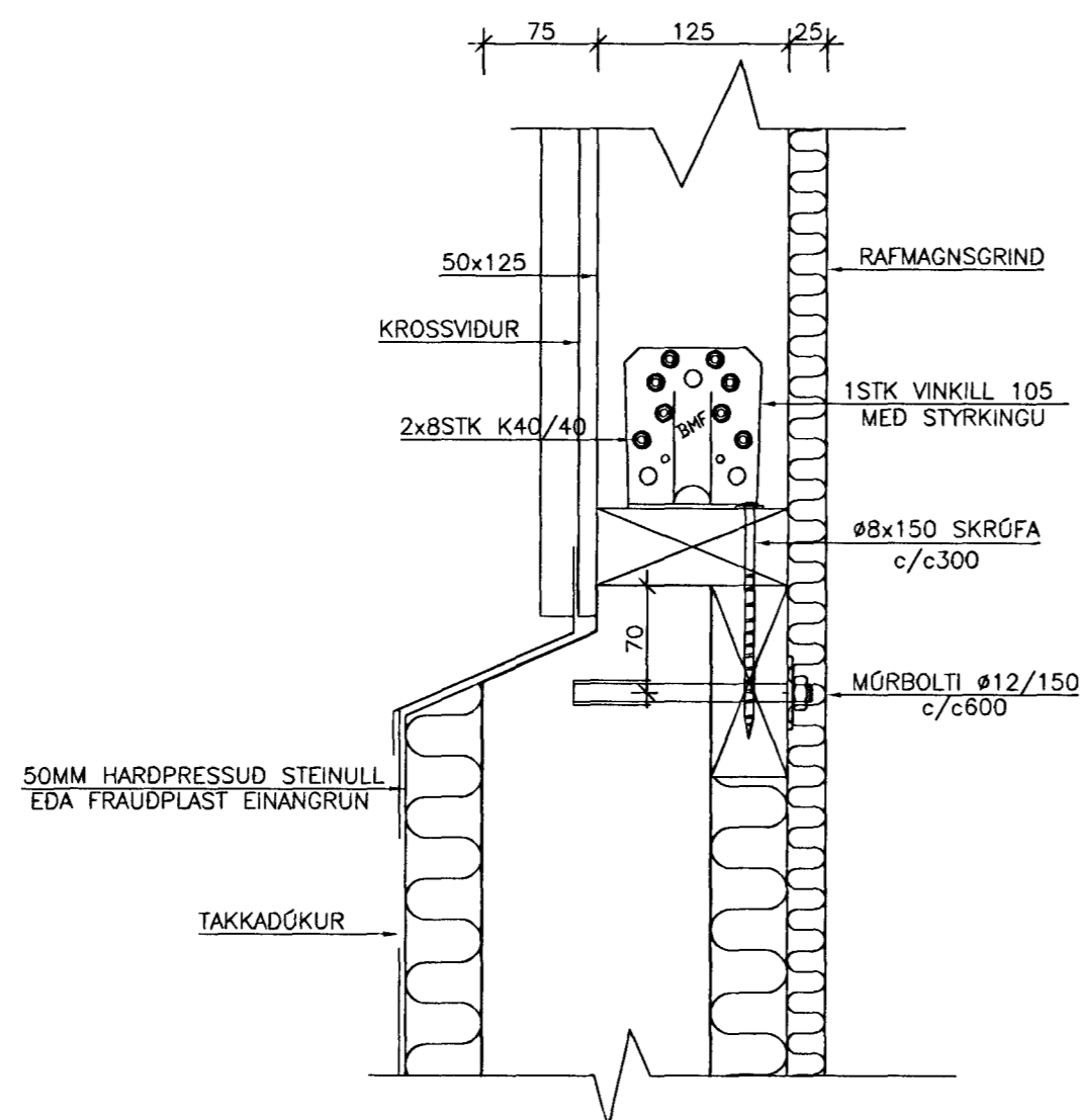
SNIÐ 11 1/5 B02&03
