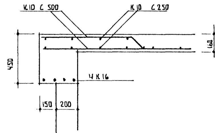
SNID I BITA YFIR DYRUM MK 1:20
