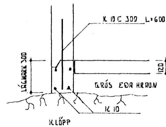
SNID I SÖKKLA MK 1:20
