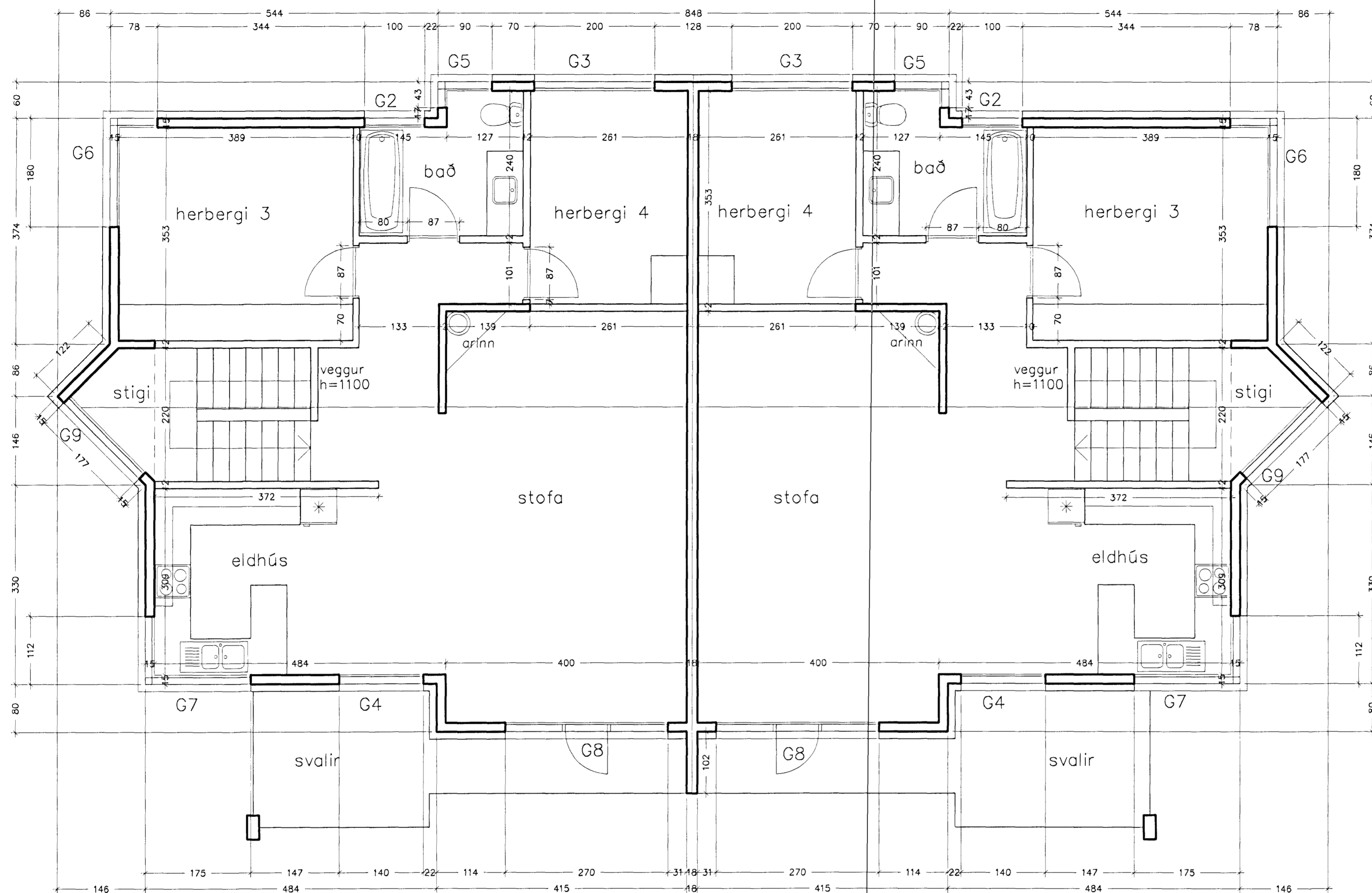
Grunnmynd 2.hæð 1:50
