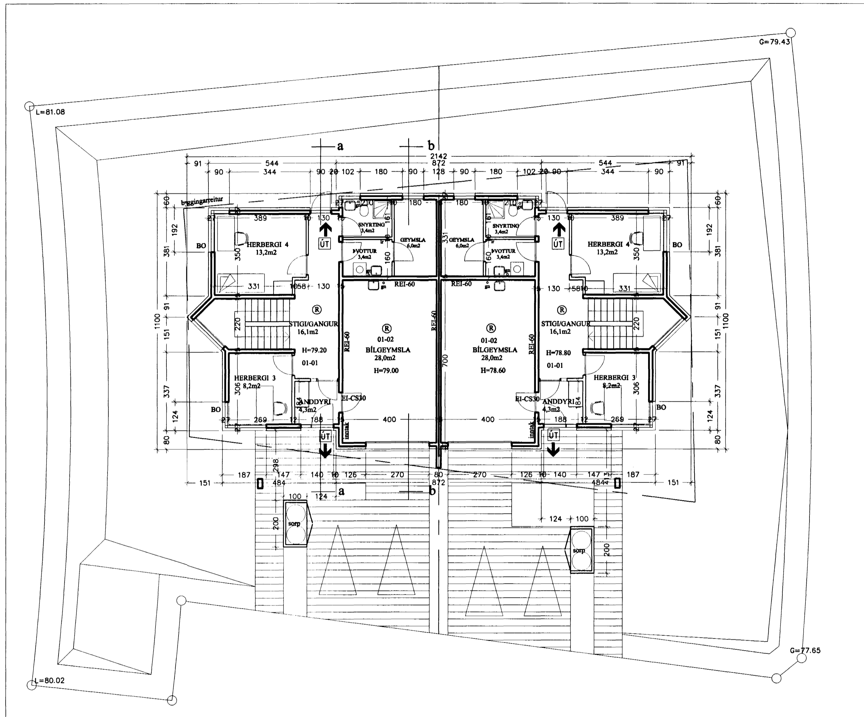
Grunnmynd 1.hæð 1:100
