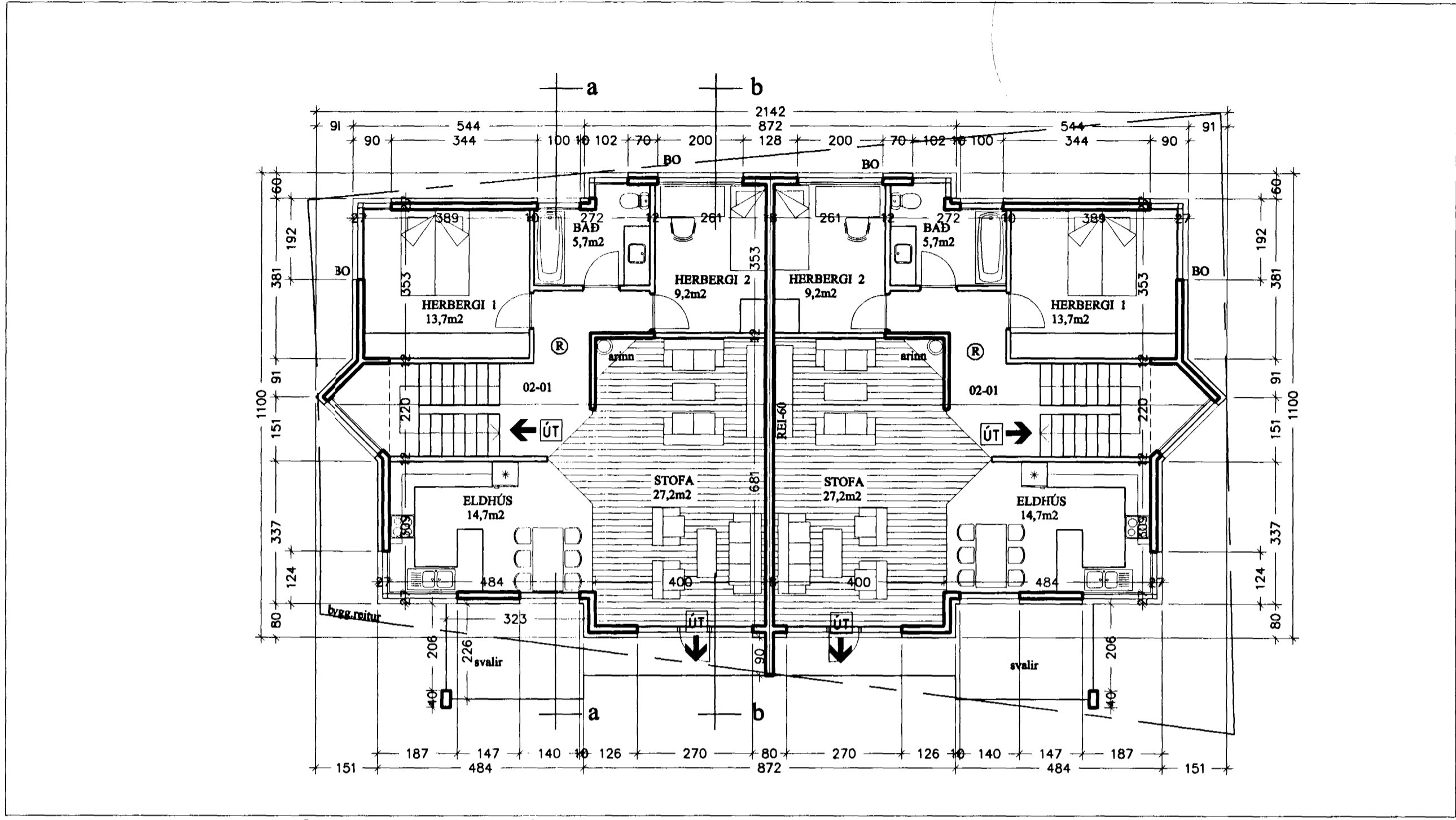
Grunnmynd 2.hæð
