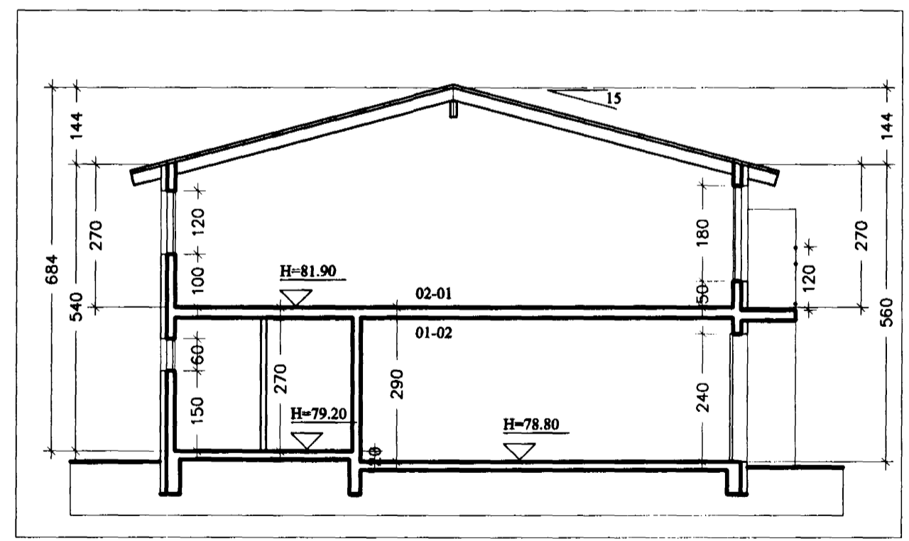
Sneiðing b-b 1:100
