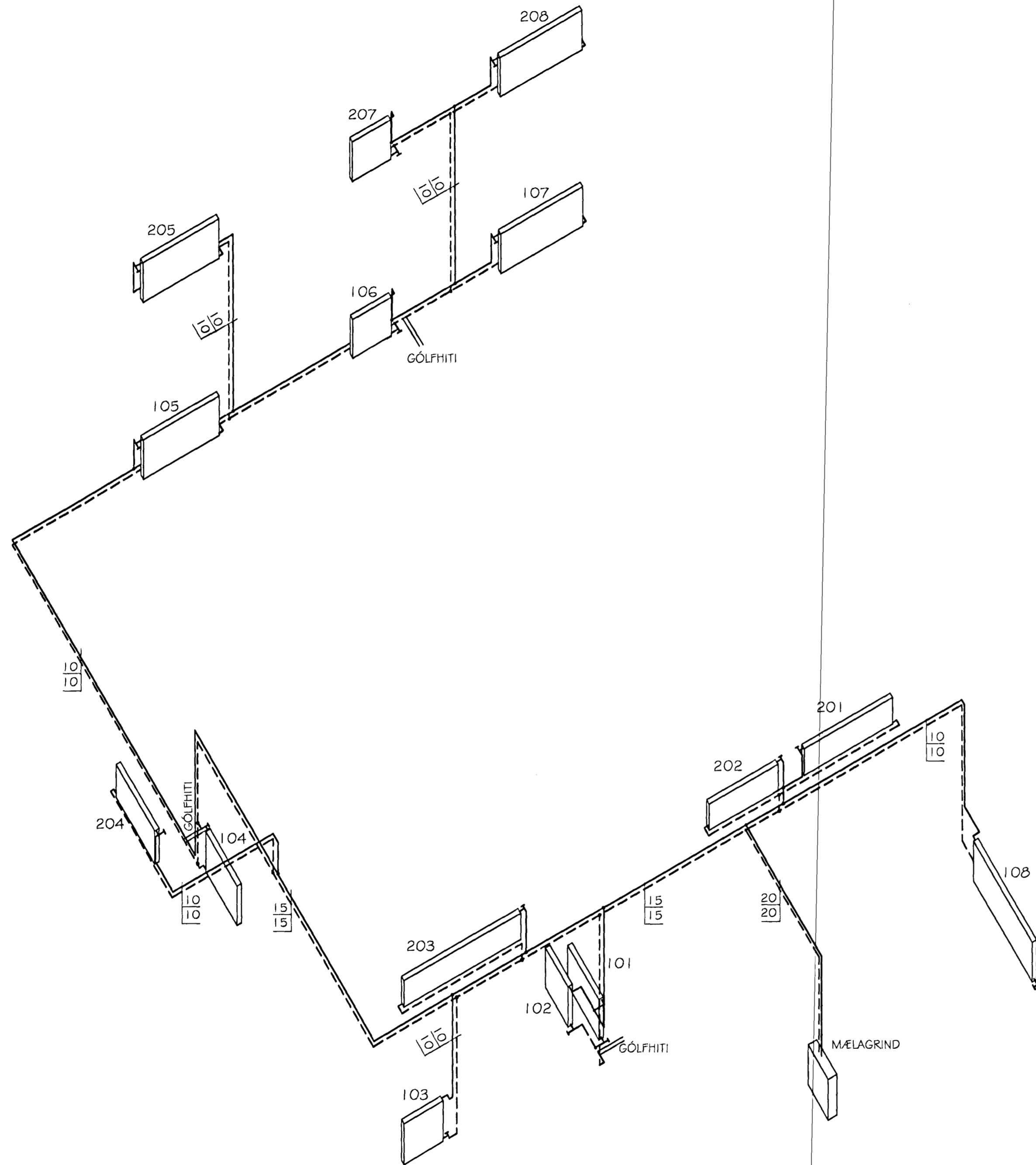
GAUKSÁS 13 HITALAGNIR RÚMMYND MKV. 1:50
