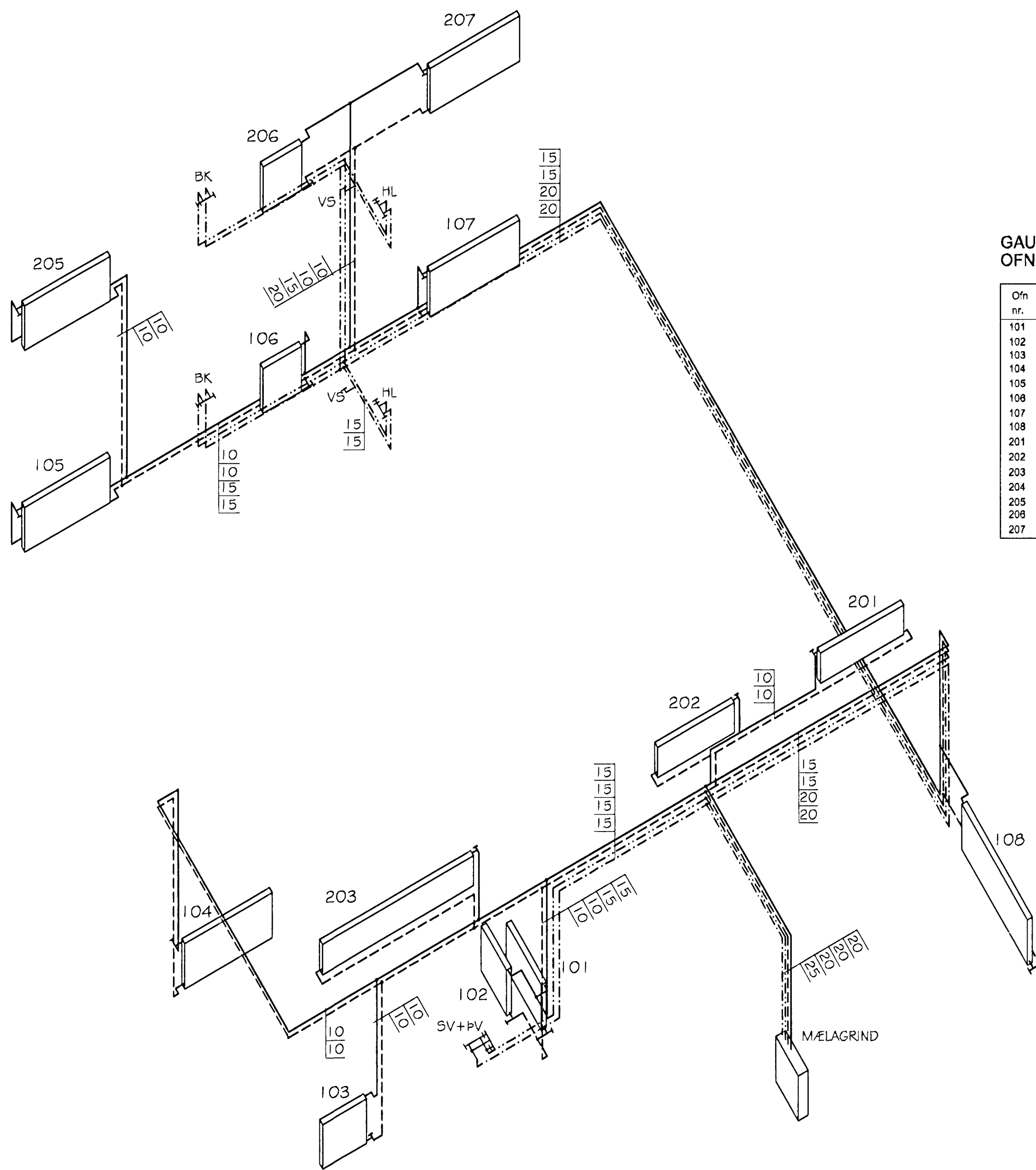
GAUKSÁS 15 NEYSLUVATNS- OG HITALAGNIR RÚMMYND MKV. 1:50
