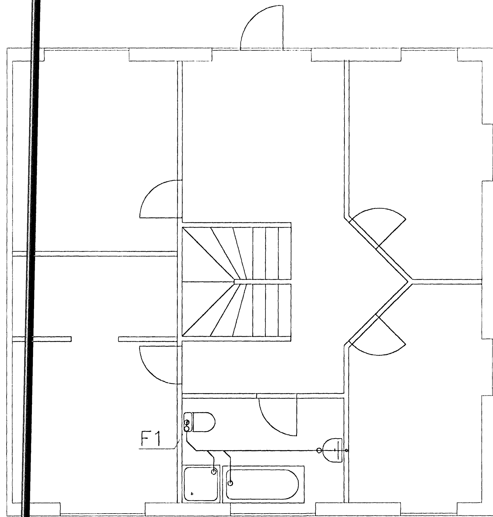
GRUNNMÝND 1:50
