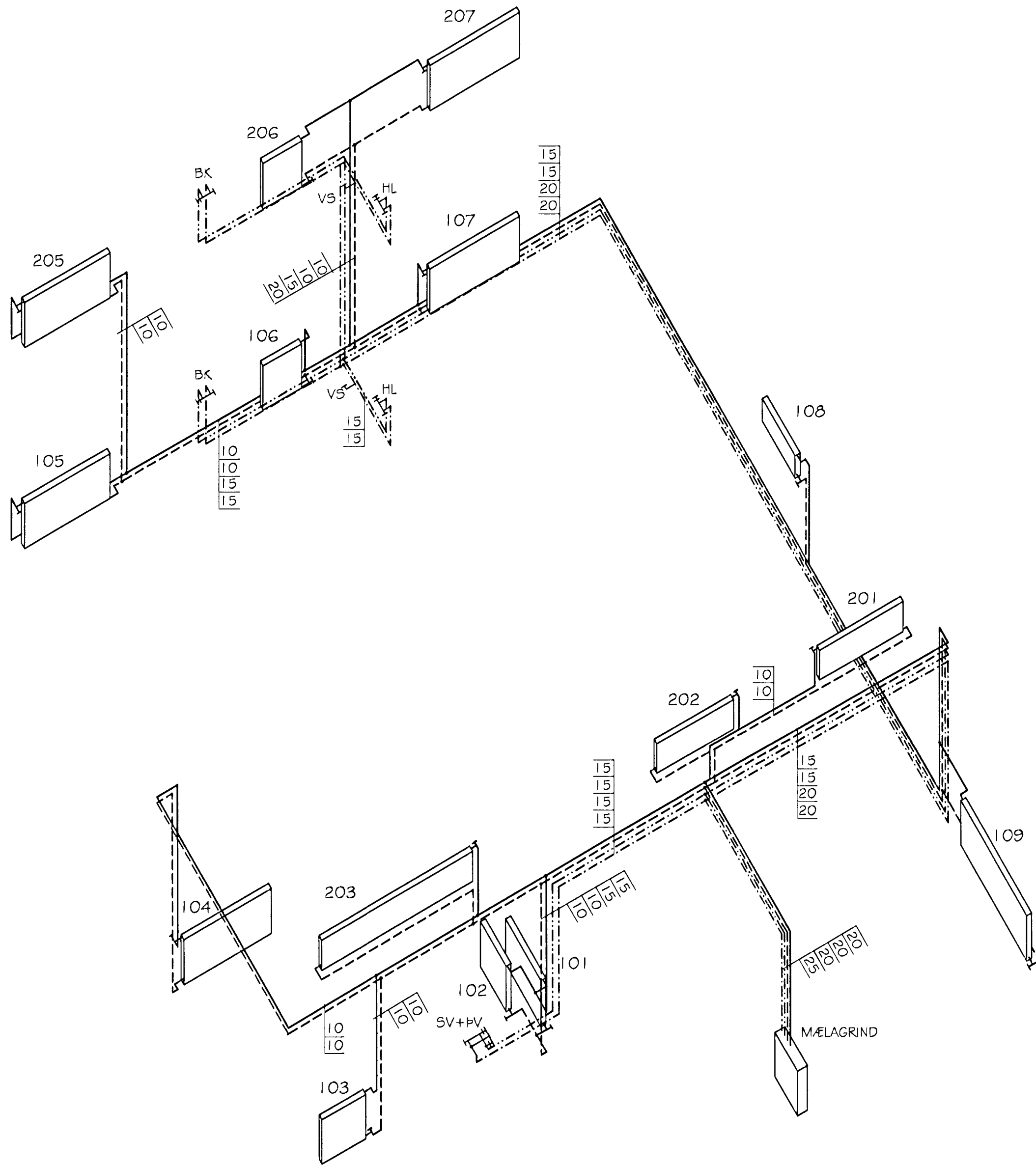
GAUKSÁS 17 NEYSLUVATNS- OG HITALAGNIR RÚMMYND MKV. 1:50
