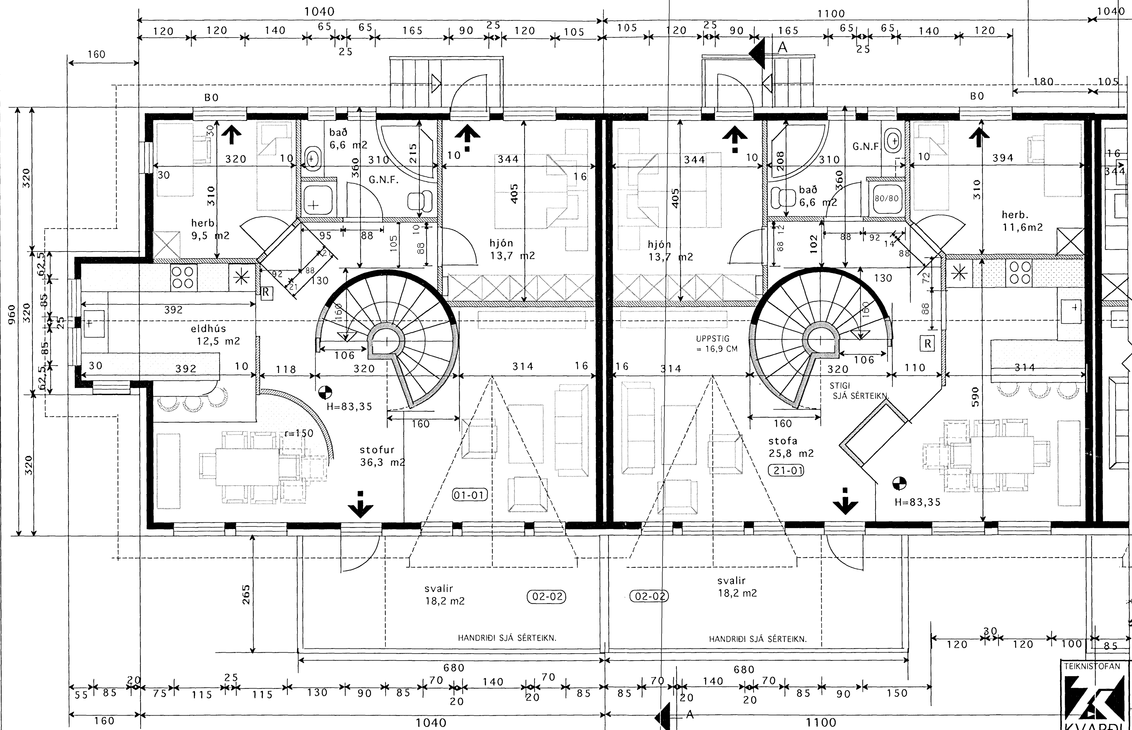
GRUNNMYND 2 HÆÐ 1:50
