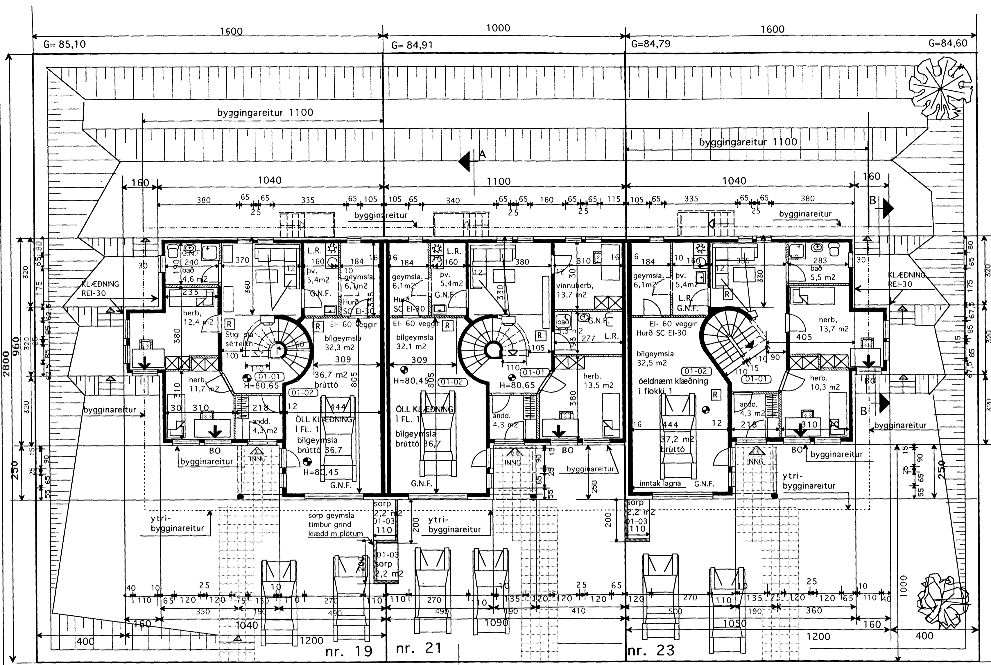
GRUNNMYND 1 HÆÐ 1:100 NÁNARI MÁLSETNING SJÁ TEIKN. V-1 1:50
