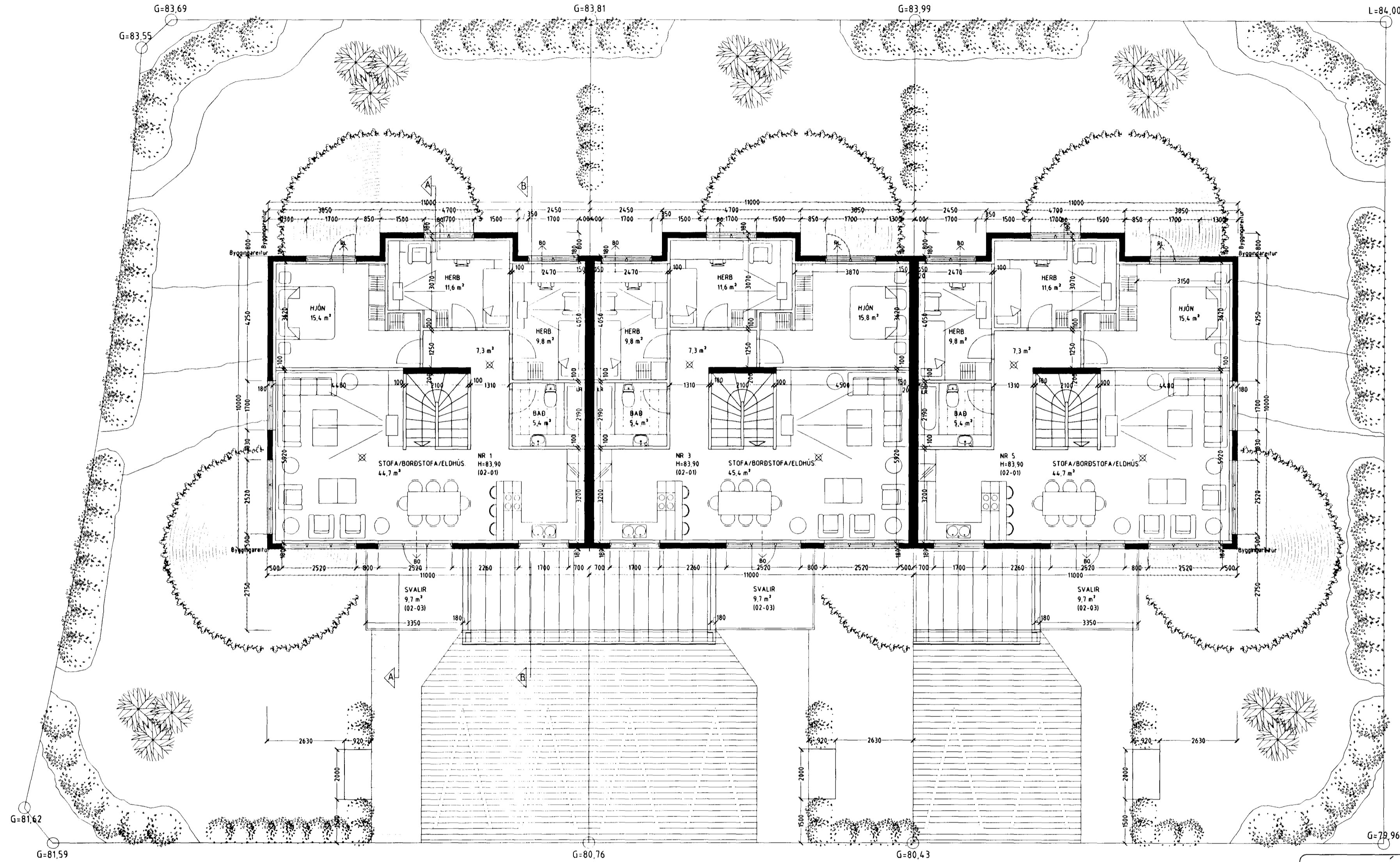
GRUNNMYND 2 HÆÐ. M. 1:100
