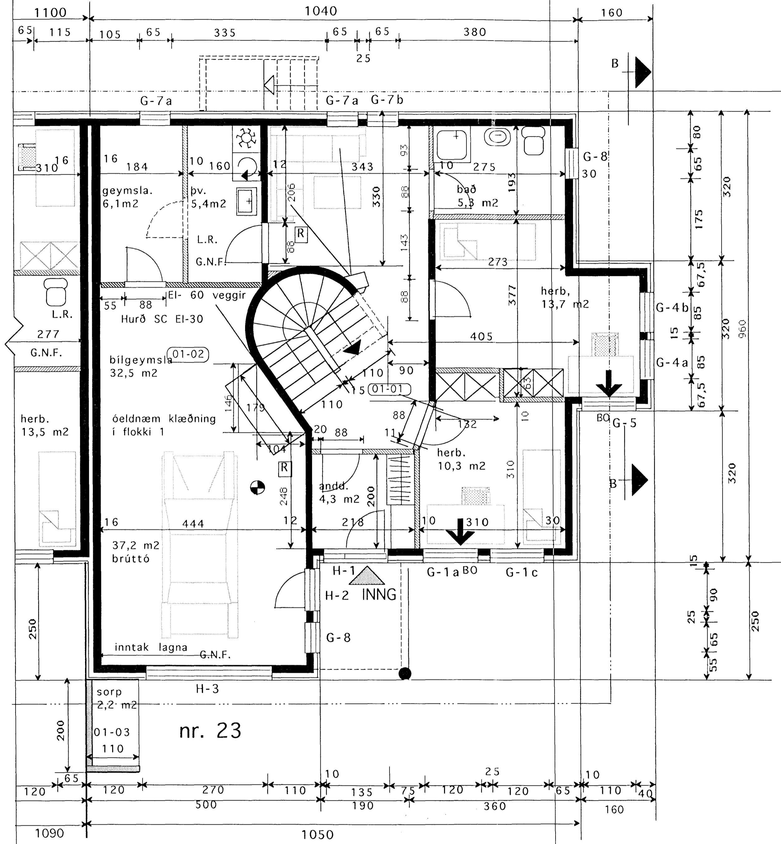
GRUNNMYND 1 HÆÐ 1:50
