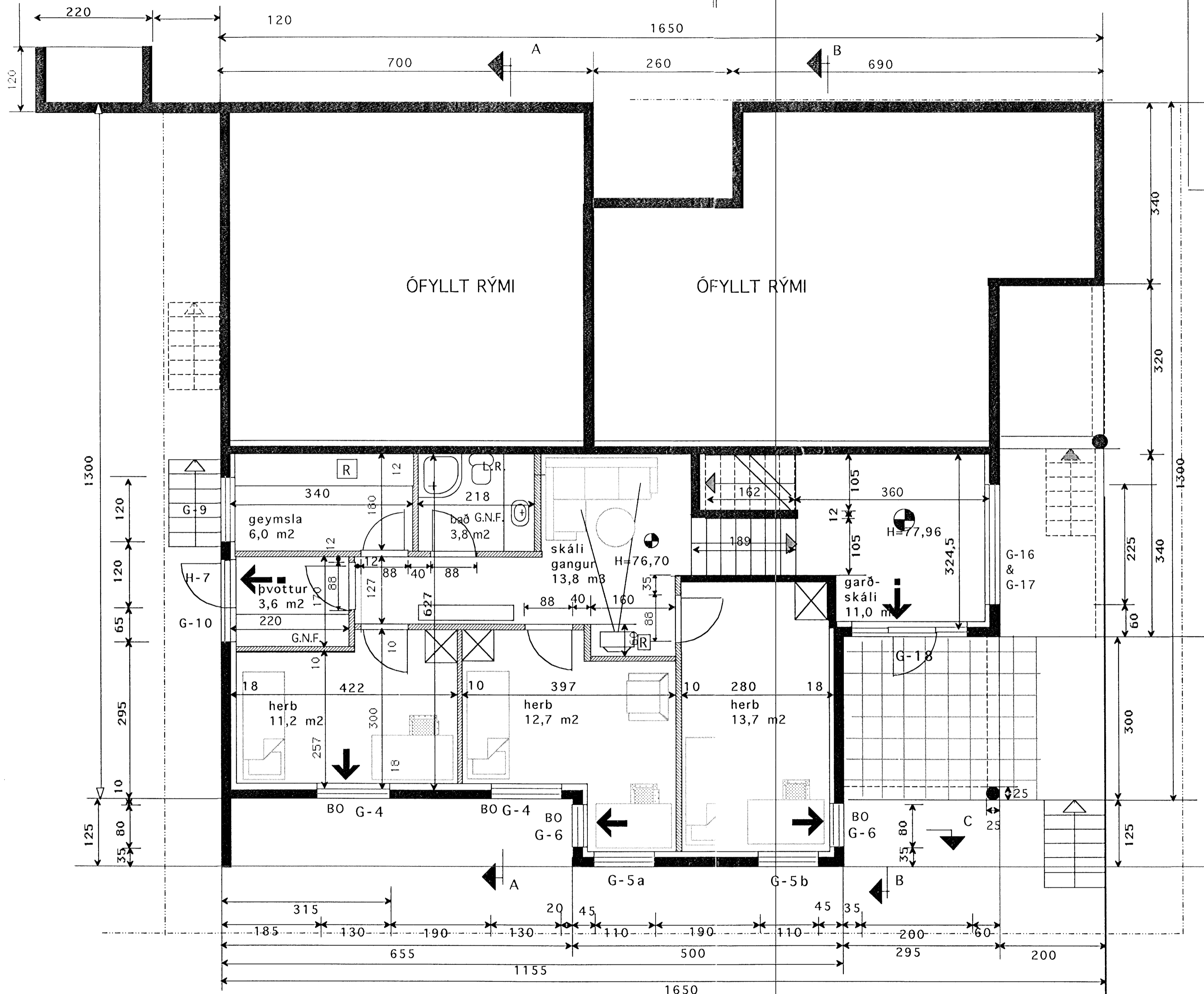
GRUNNMYND 1 HÆÐ
