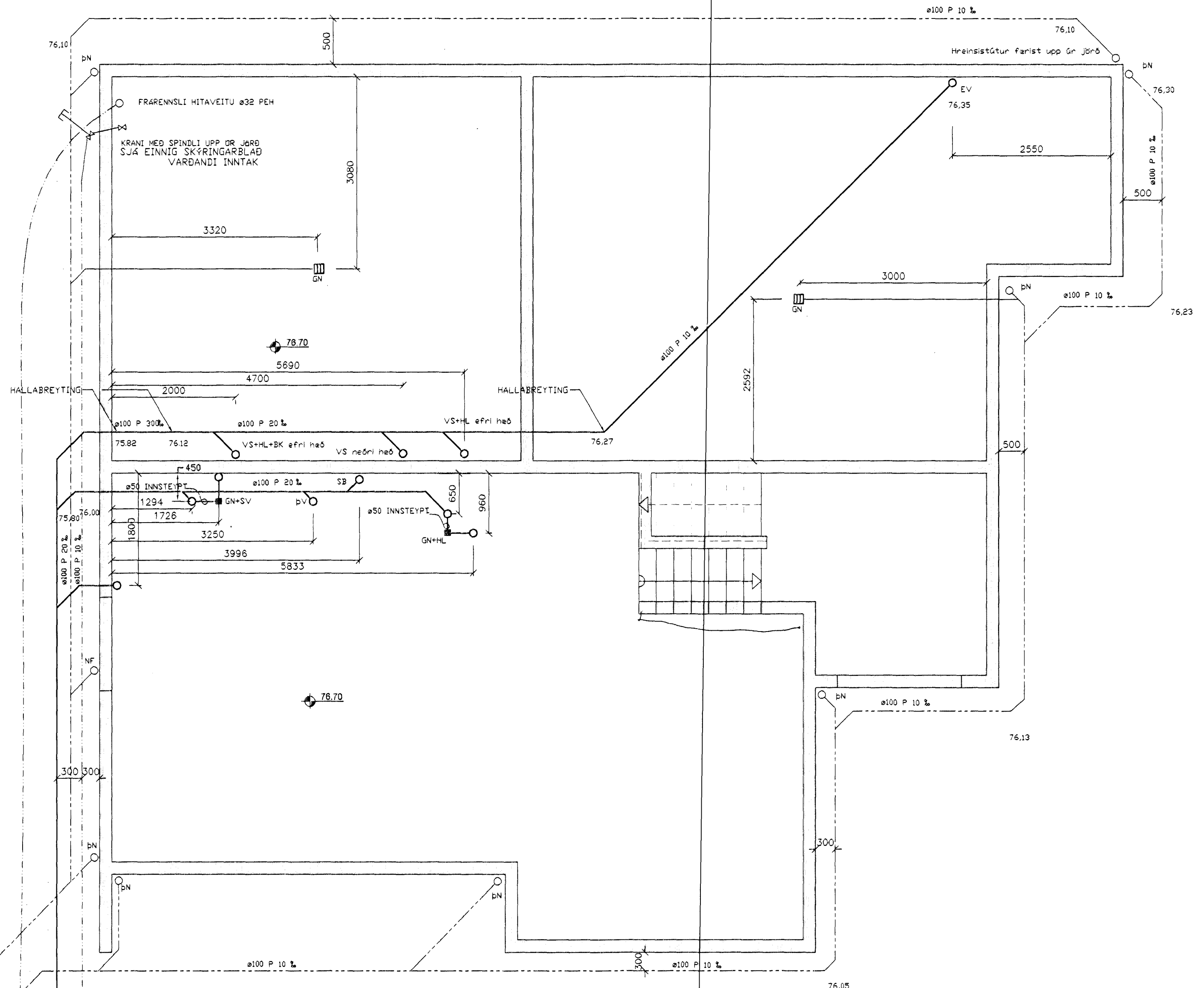
GRUNNMYND LAGNA Í SÖKKLI 1:50
