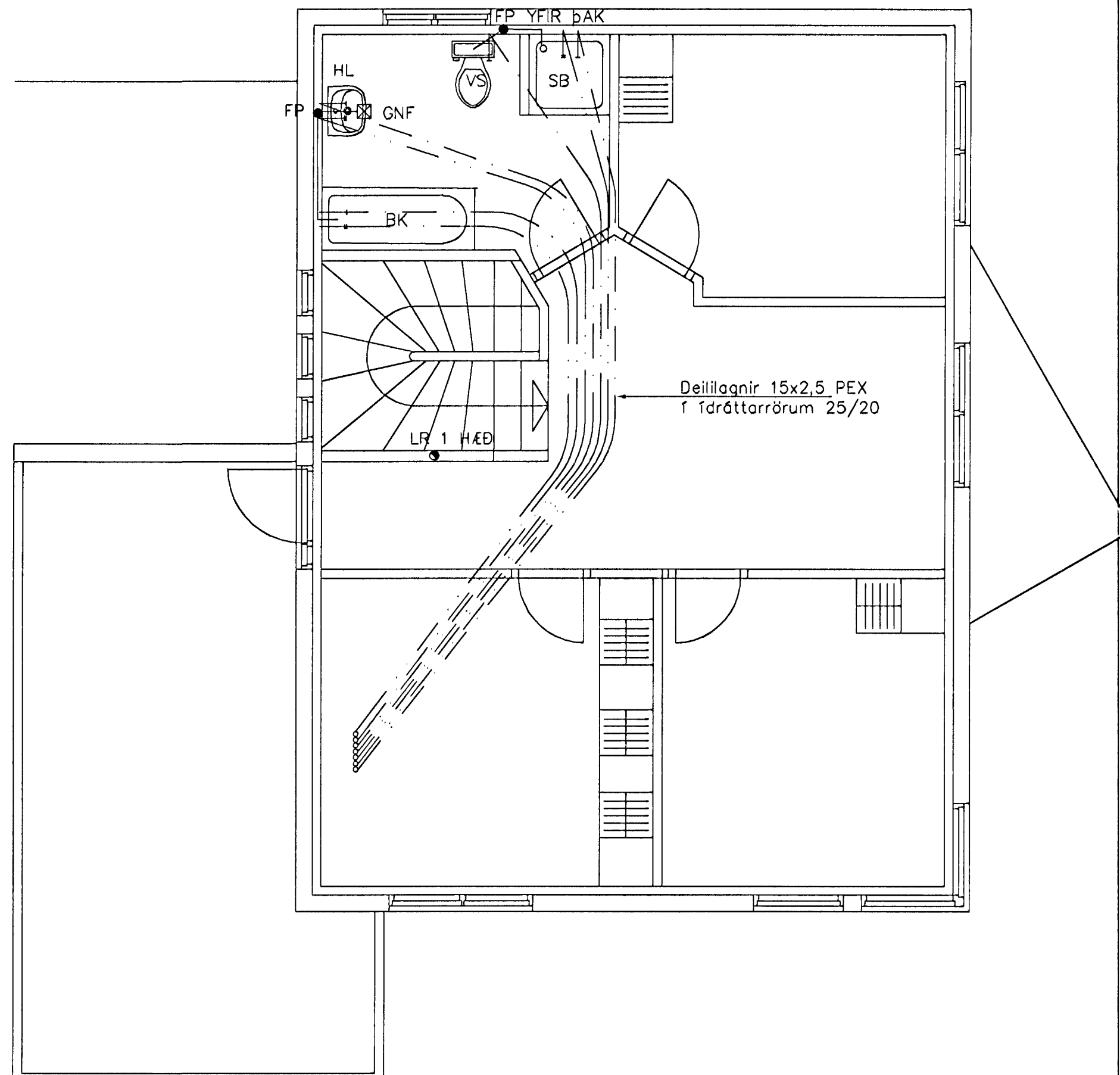
GRUNNMYND 2 HÆÐAR 1:50
