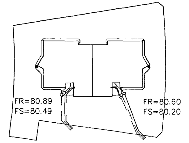
AFSTÖÐUMYND 1:500
