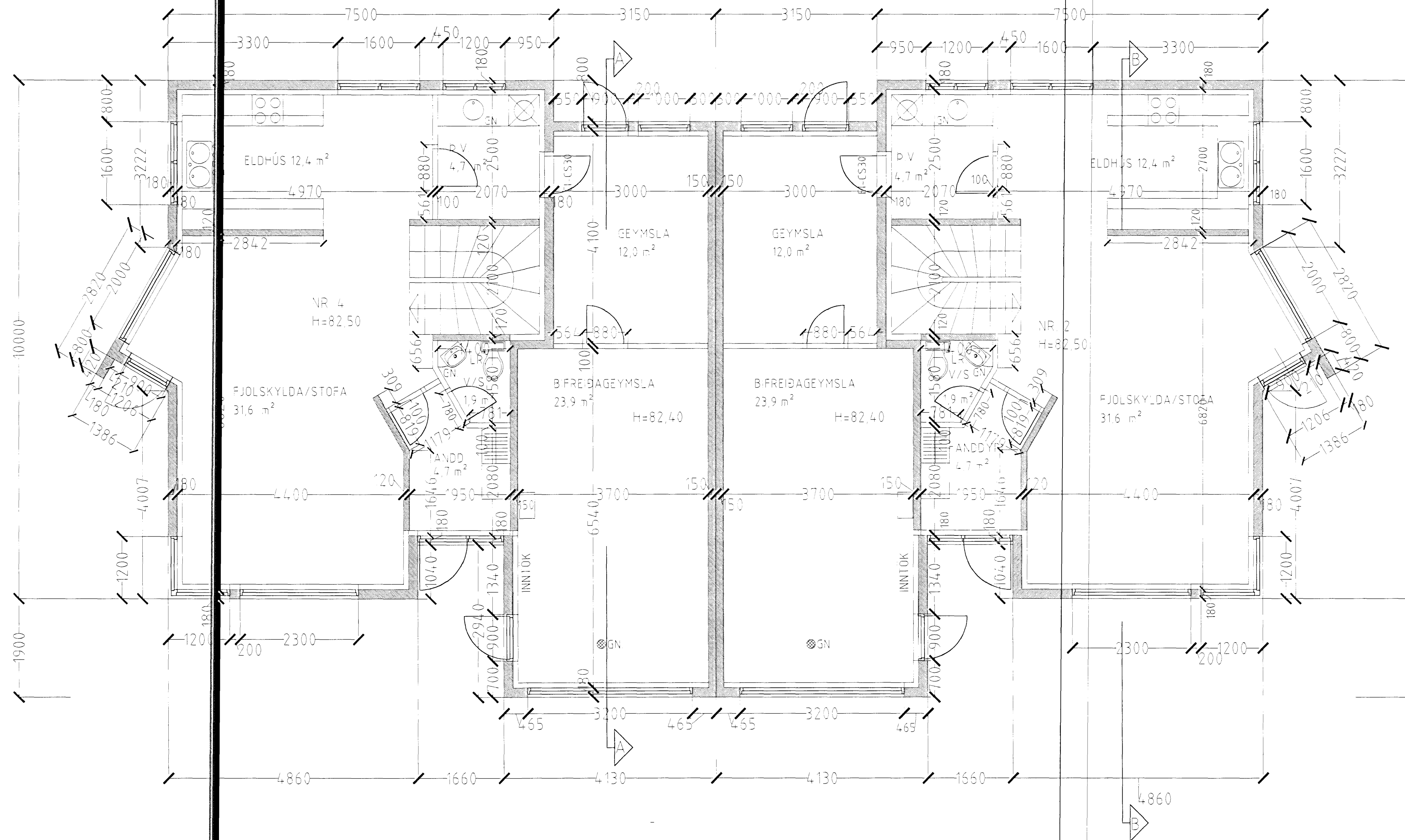
GRUNNMYND 1 HÆÐ MKV. 1:50.
