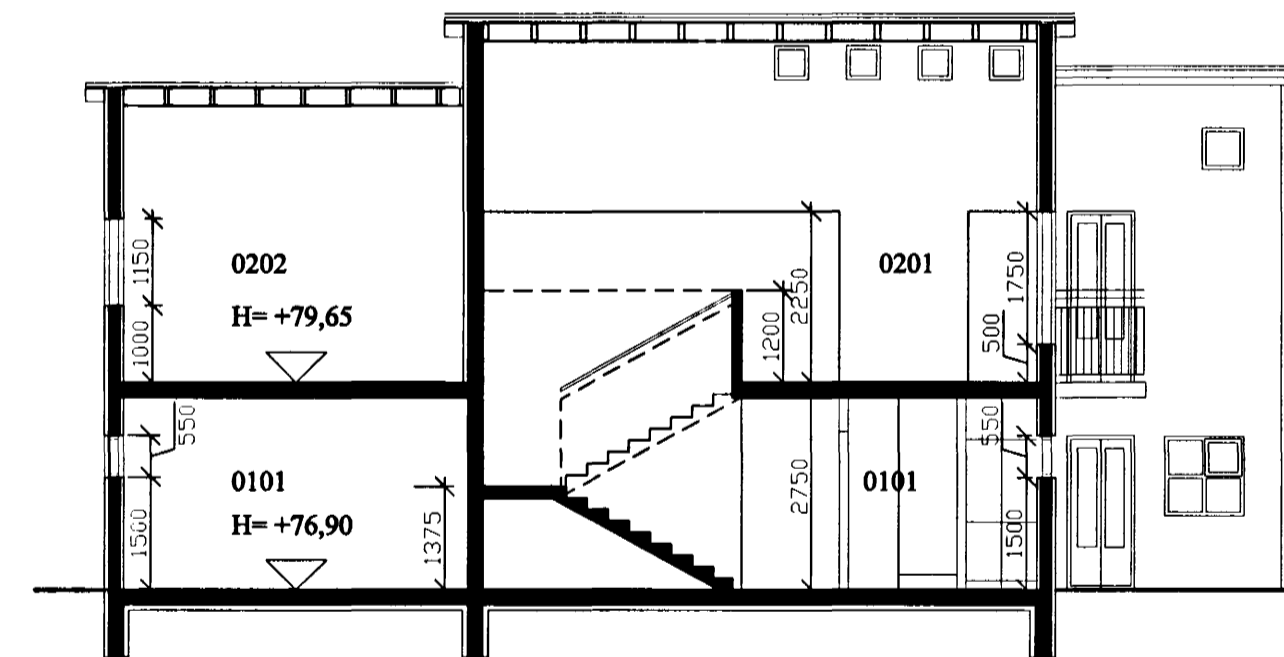
Skurður b-b 1:100
