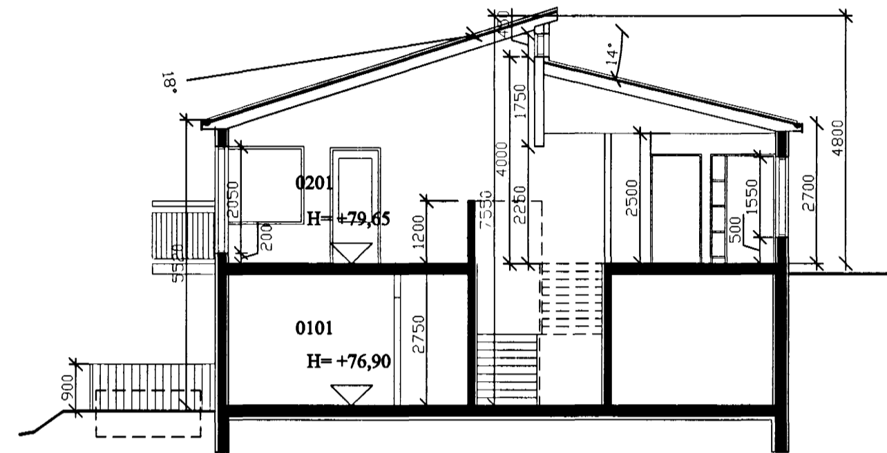
Skurður a-a 1:100
