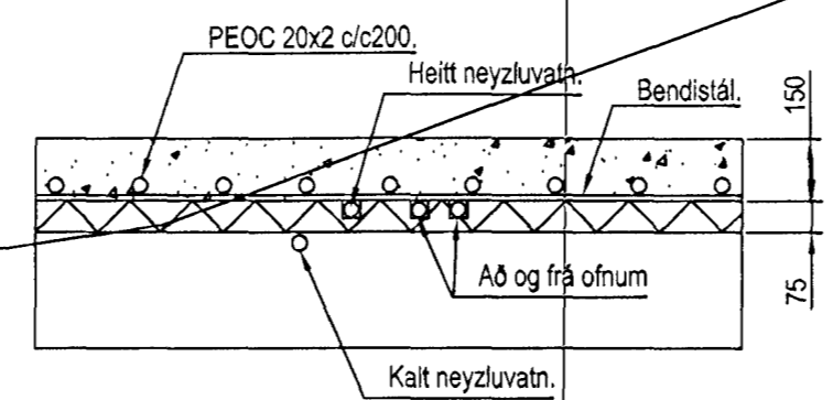
Snið í gólfplötu/staðsetning á pípum. Mk 1:20.
