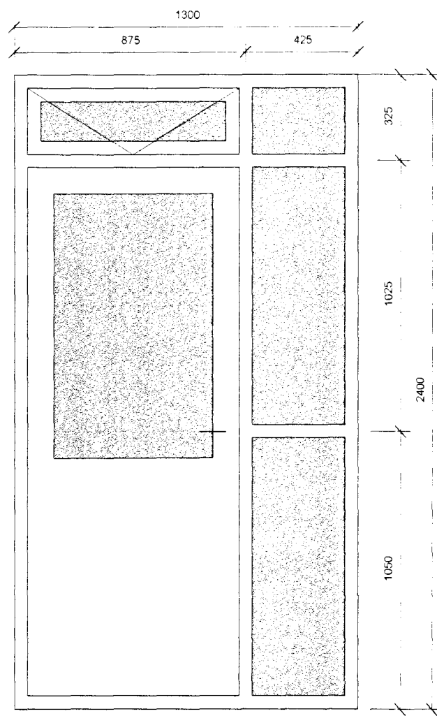
GH-2 1stk Þvottahús. 2400 mm í efribrún frá endanlegu gólfi.
