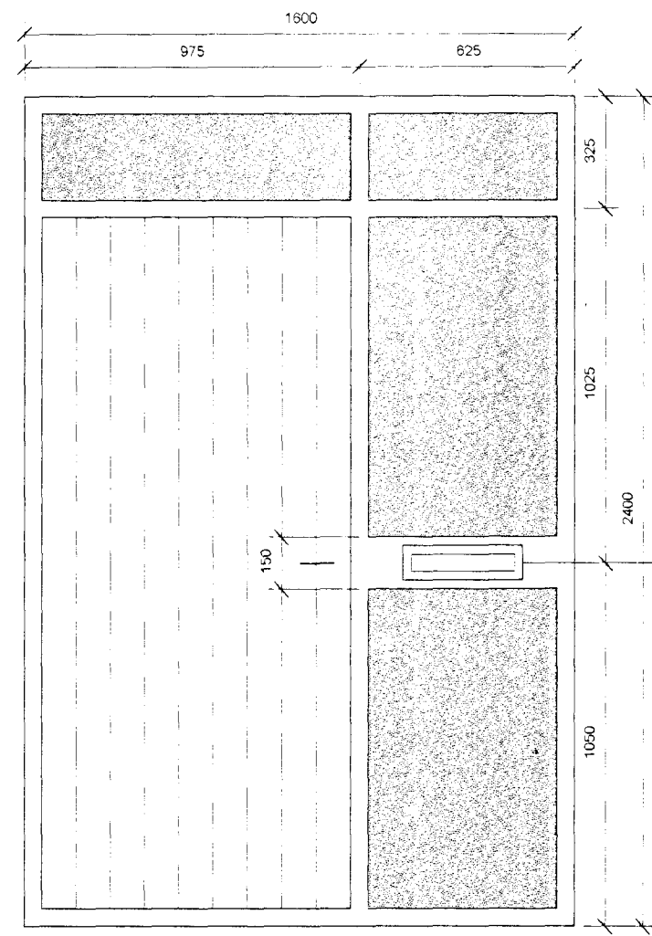
GH-1 1stk Útidyráhurð. 2400 mm í efribrún frá endanlegu gólfi.
