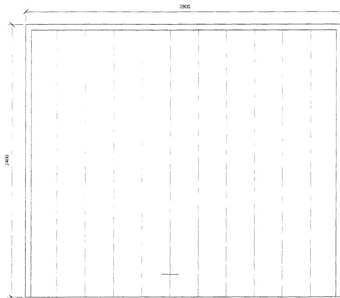
H-1 1stk Bílskúrshurð. 2400 mm í efribrún frá endanlegu gólfi.
