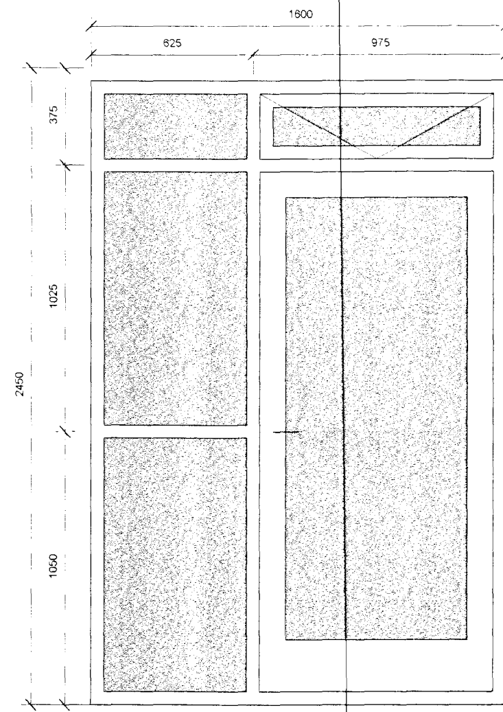
GH-3 1stk Svalahurð. 2400 mm í efribrún frá endanlegu gólfi.
