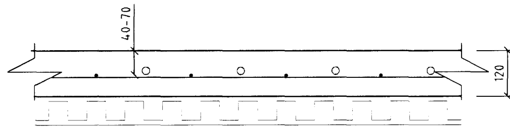
Dversnið 1:10
