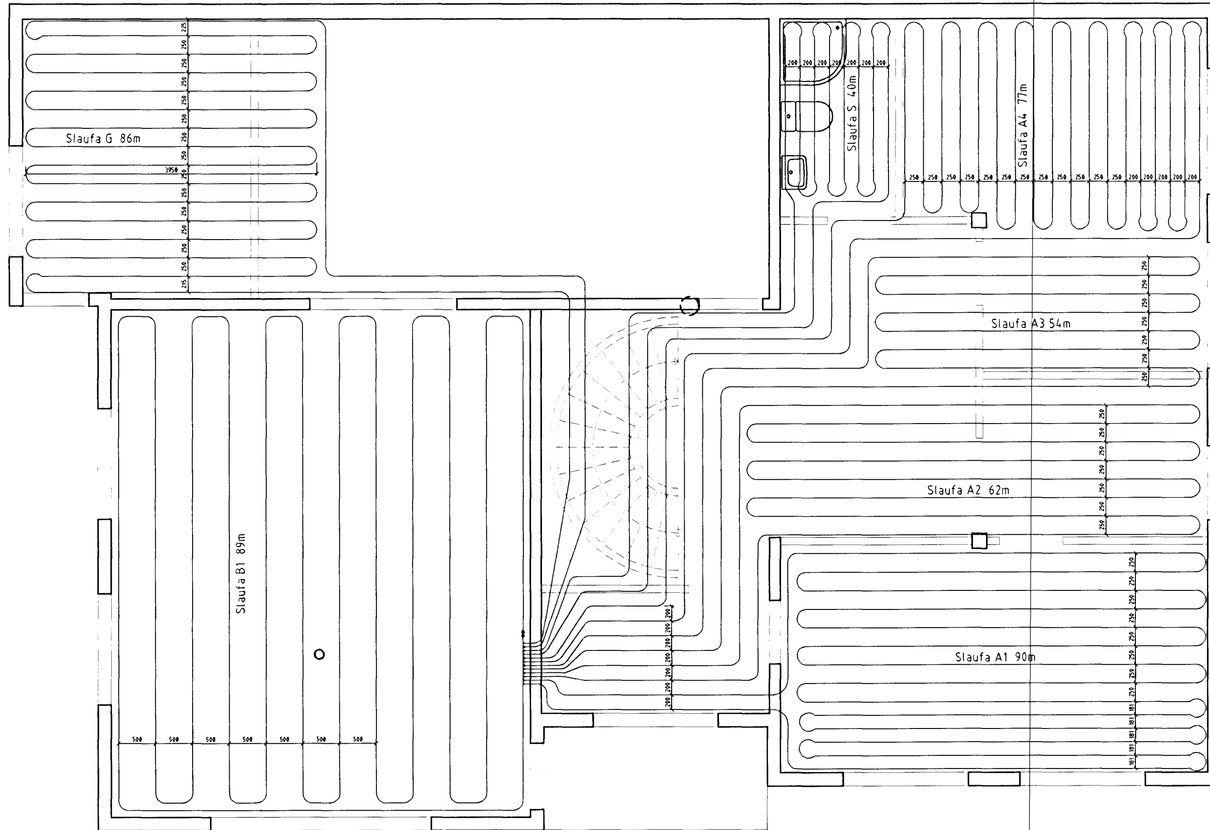
Grunnmynd 1:50
